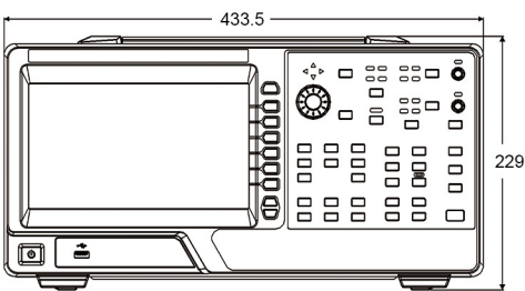
PA2000mini机械尺寸图 (正面)
