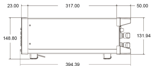
PA323/PA323H/PA333H/PA333H-2K/PV300型功率计 机械尺寸图 (侧面)
