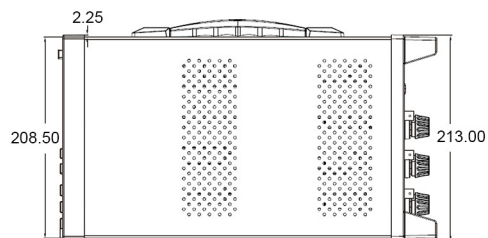
PA323/PA323H/PA333H/PA333H-2K/PV300型功率计 机械尺寸图 (俯视)
