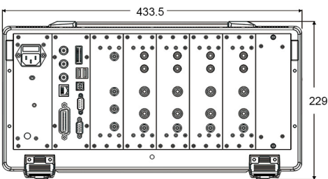
PA2000mini机械尺寸图 (背面)
