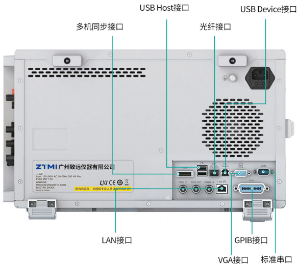
PA8000、PA5000H、PA6000H 接口图
