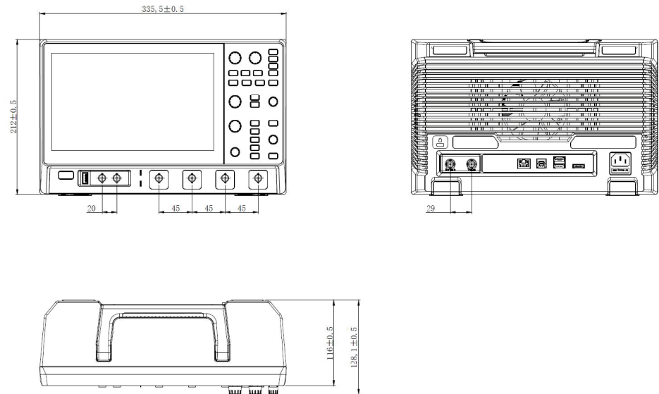
图 4.1 ZUS5000 示波器尺寸图
