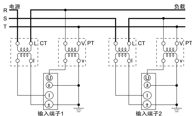
图 4.42 三相 3 线制(3P3W)、使用 PT/CT 时的接线举例
