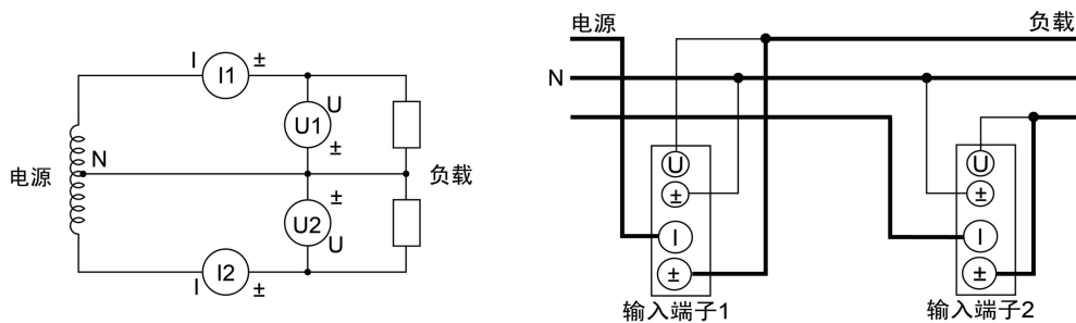
图 4.38 单相 3 线制(1P3W), 测量仪表的接线
