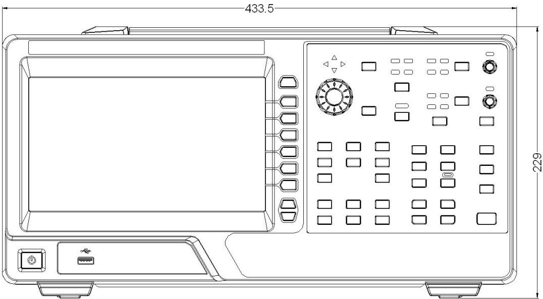
图 7.2 尺寸图 2
