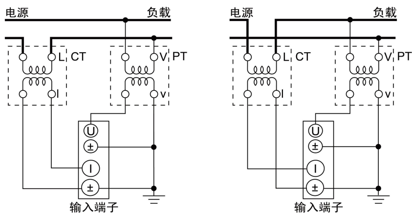
图 4.36 单相 2 线制(1P2W)，使用 PT/CT 时的接线举例
