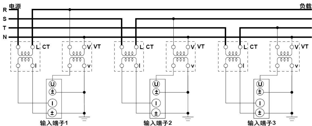
图 4.48 三相 4 线制(3P4W)、使用 PT/CT 时的接线举例
