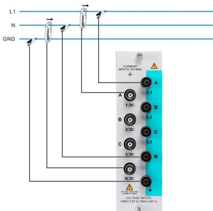
图 4.50 1P2W-Neutral
