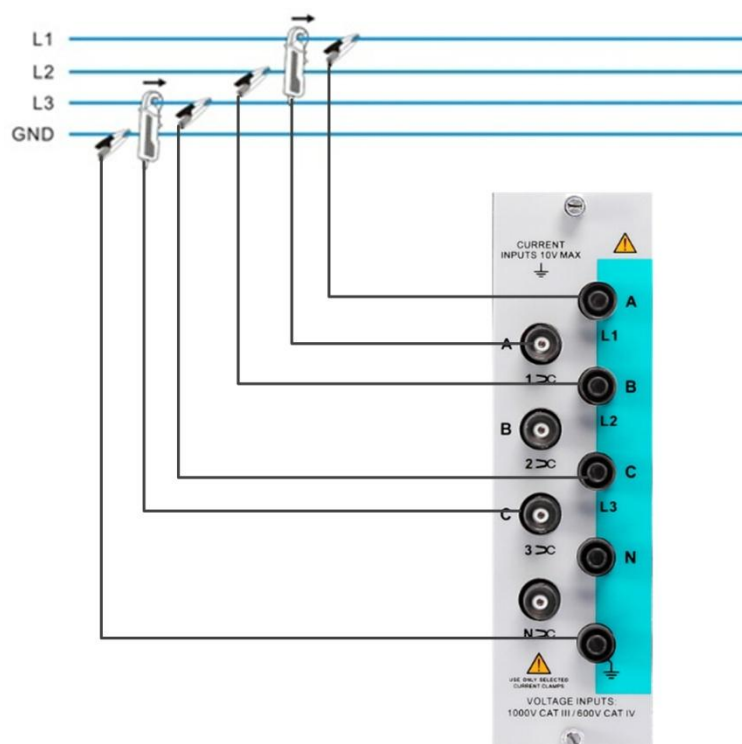
图 4.52 3P3W-2-Element
