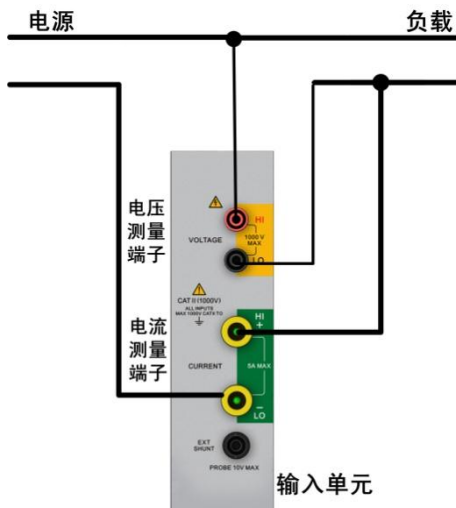
图 4.37 1P2W 下光伏逆变器综合测试仪接线实例
