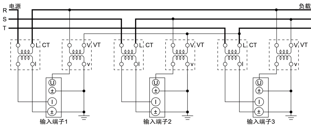
图 4.45 三相 3 线制 (3 电压 3 电流表法)，使用 PT/CT 的接线
