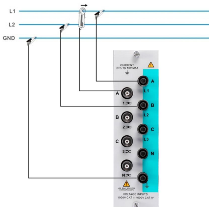
图 4.51 1P2W-No Neutral
