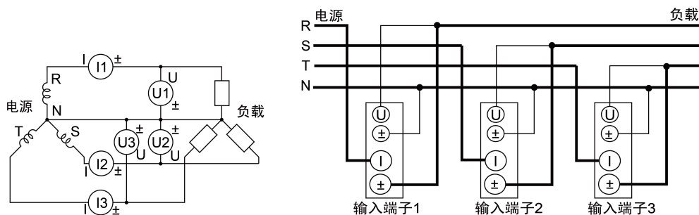
图 4.47 三相 4 线制下的测量仪表接线
