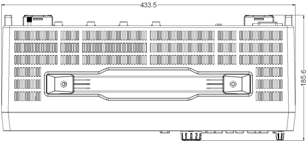
图 7.1 尺寸图 1
