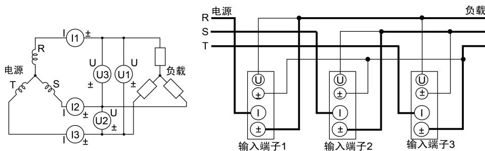
图 4.44 三相 3 线制 (3 电压 3 电流表法)，测量仪表接线
