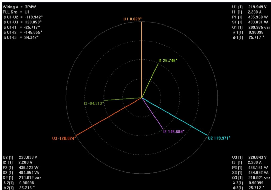
图 2.13 向量显示
