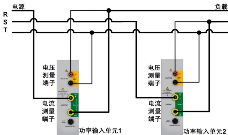
图 4.43 3P3W 下光伏逆变器综合测试仪接线示例
