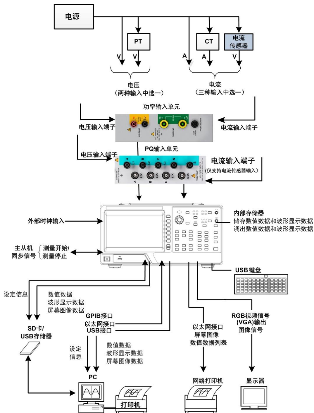
图 1.2 应用系统
