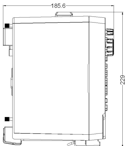
图 7.3 尺寸图 3
