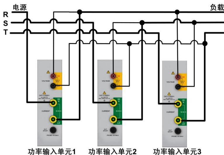
图 4.46 3P3W (3 电压 3 电流表法) 下光伏逆变器综合测试仪接线示例
