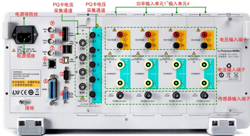
图 3.14 后面板说明
