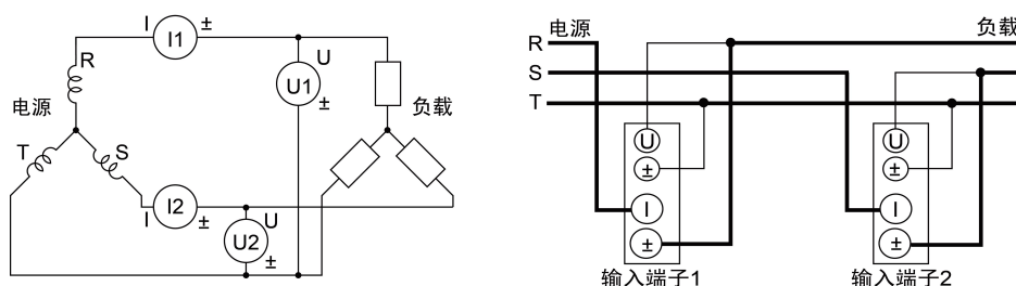
图 4.41 三相 3 线制、测量仪表的接线
