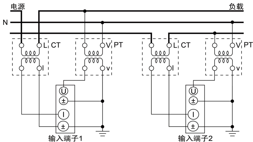
图 4.39 单相 3 线制(1P3W)、使用 PT/CT 时的接线举例
