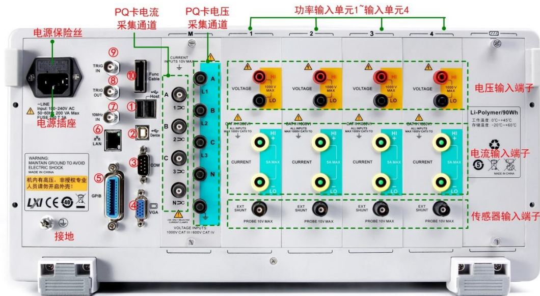
图 2.19 信号输入单元
