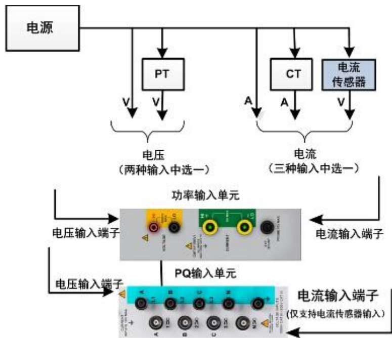
图 2.20 输入信号到输入单元
