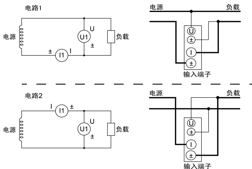
图 4.35 单相 2 线制(1P2W)，测量仪表的接线
