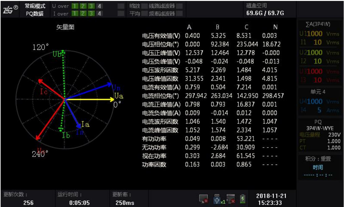
图 2.18 PQ 数据
