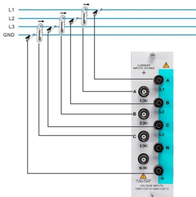
图 4.53 3P3W-IT 和 3P3W-Delta
