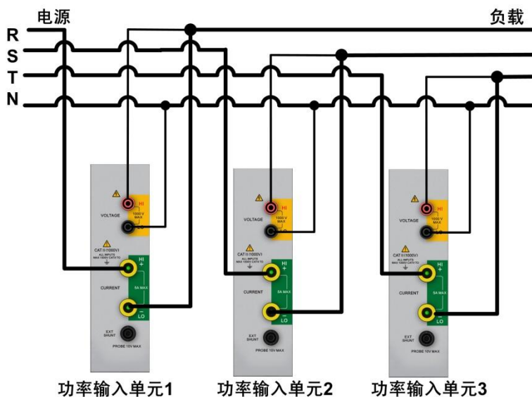
图 4.49 三相 4 线制接线实例
