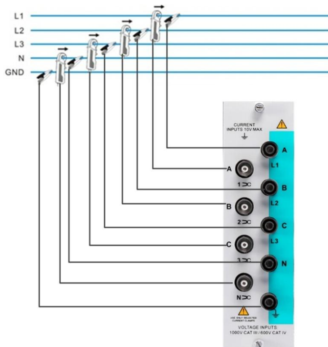
图 4.54 3P4W-High Leg 和 3P4W-WYE
