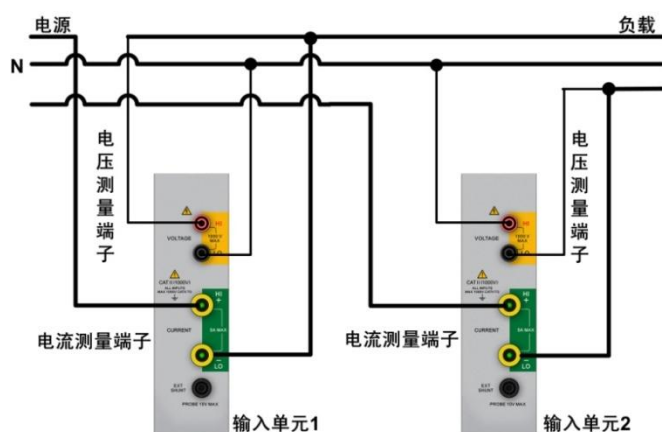
图 4.40 1P3W 下光伏逆变器综合测试仪接线实例
