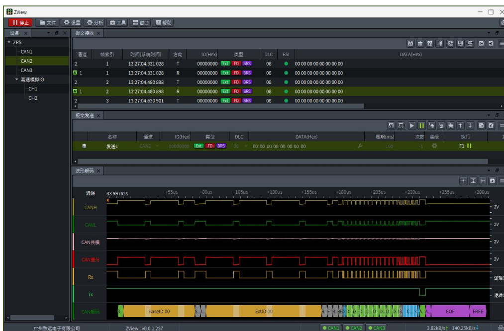
图 4.8 报文窗口
