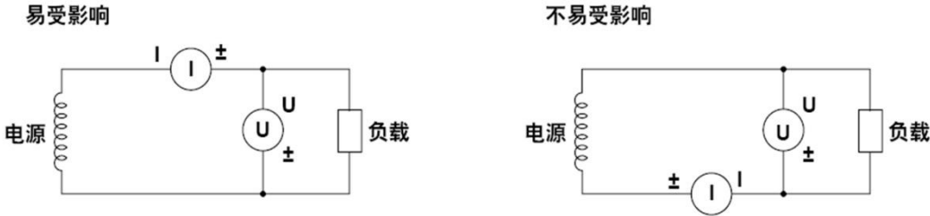
图 4.33 降低杂散电容对测量精度的影响
