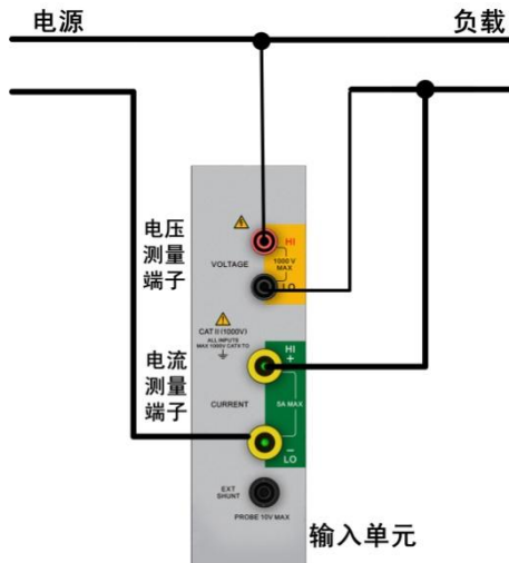
图 4.37 1P2W 下新能源汽车综合分析仪接线实例
