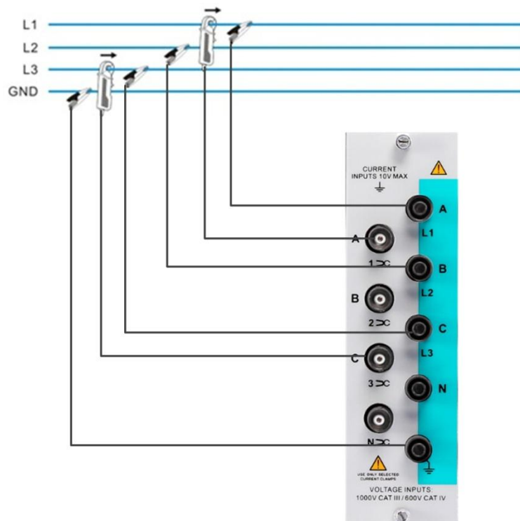
图 4.52 3P3W-2-Element
