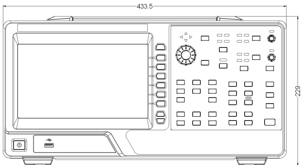
图 7.2 尺寸图 2
