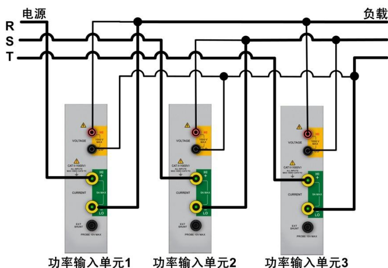
图 4.46 3P3W (3 电压 3 电流表法) 下新能源汽车综合分析仪接线示例
