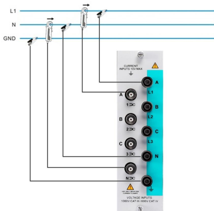
图 4.50 1P2W-Neutral
