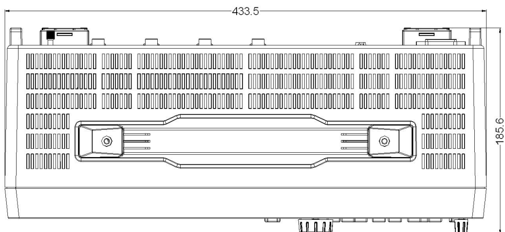
图 7.1 尺寸图 1
