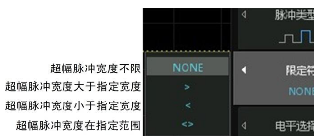
图 10.34 超幅触发的限定符
