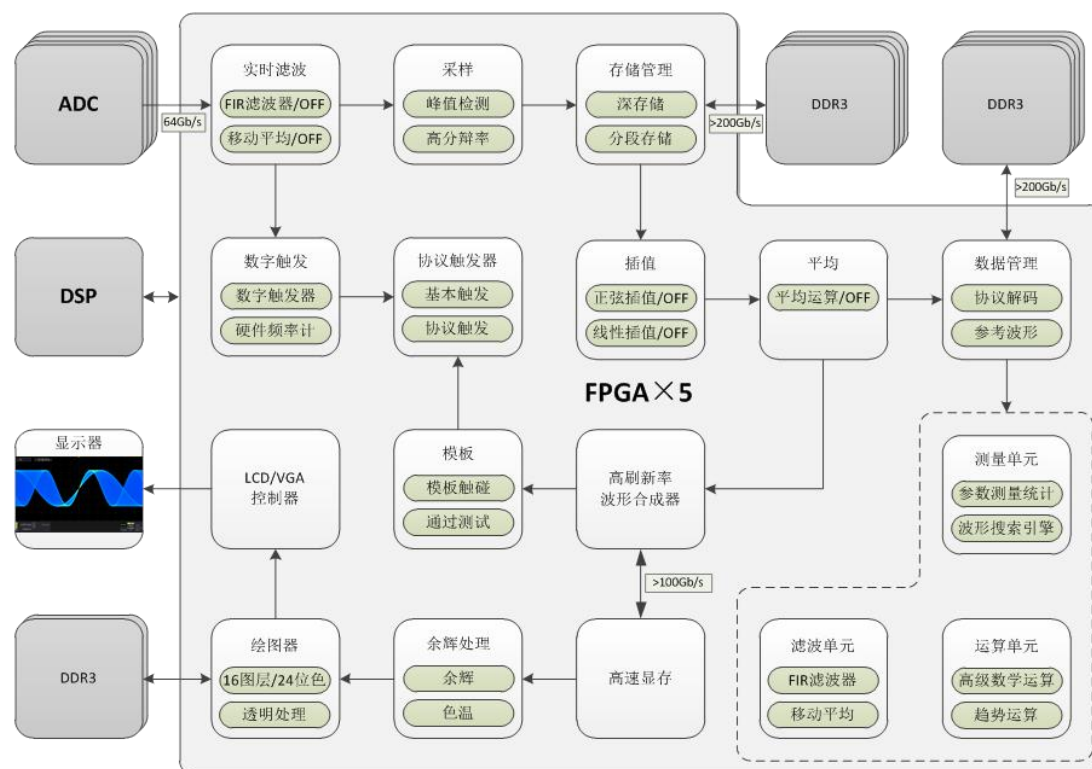
图 3.3 ZDS5000 系列示波器系统框图
