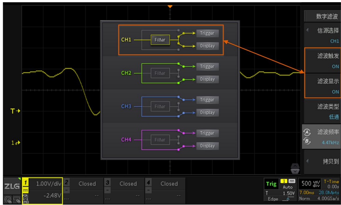
图 16.3 滤波触发和显示
