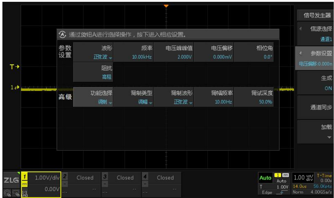
图 20.6 调制参数设置
