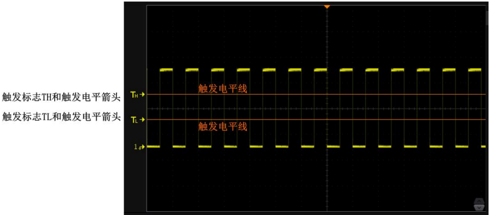
图 10.3 TH 和 TL 触发标志
