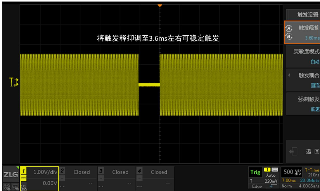
图 10.17 波形稳定显示
