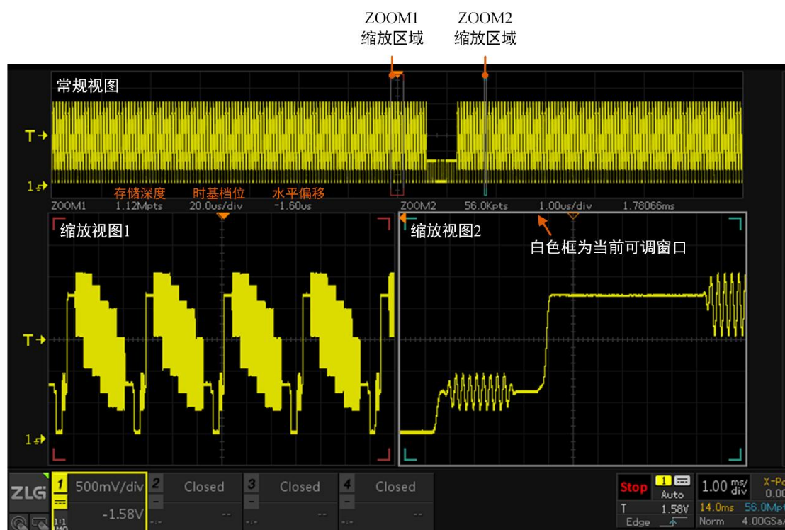
图 6.5 双 ZOOM 显示模式
