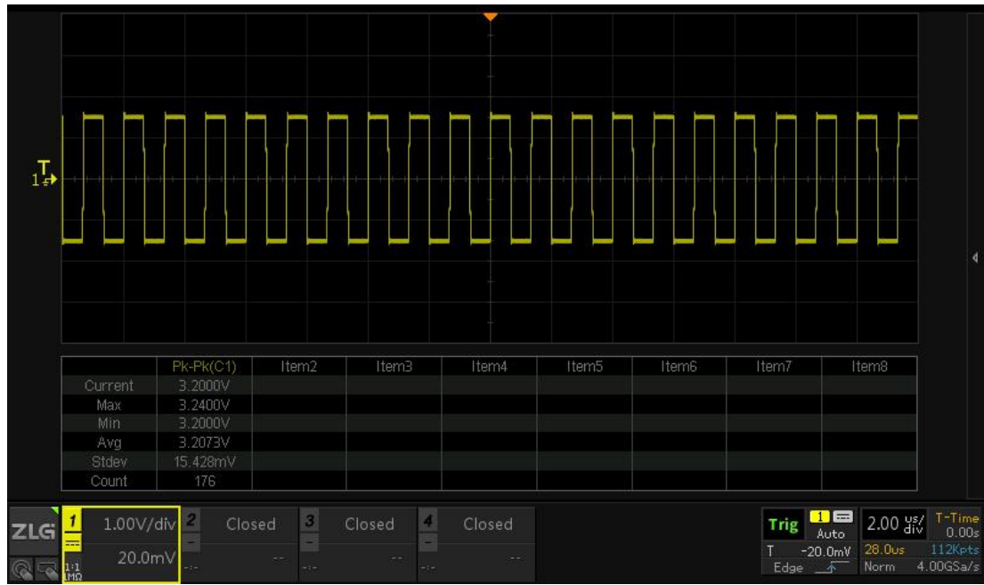
图 12.10 峰值测量结果
