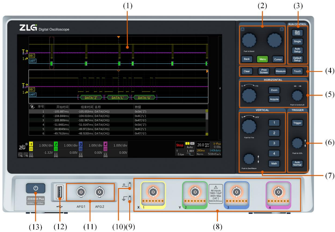
图 5.8 ZDS5054Pro 型台式示波器前面板
