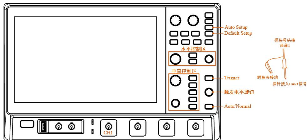
图 13.4 接入毛刺信号
