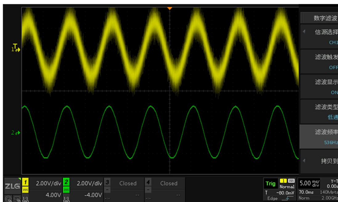
图 16.6 噪声滤波效果图
