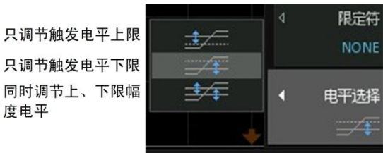
图 10.31 上限幅度电平、下限幅度电平的调节方式
