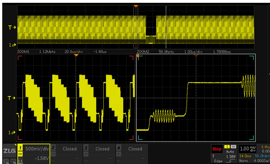
图 9.13 双 ZOOM 模式界面
