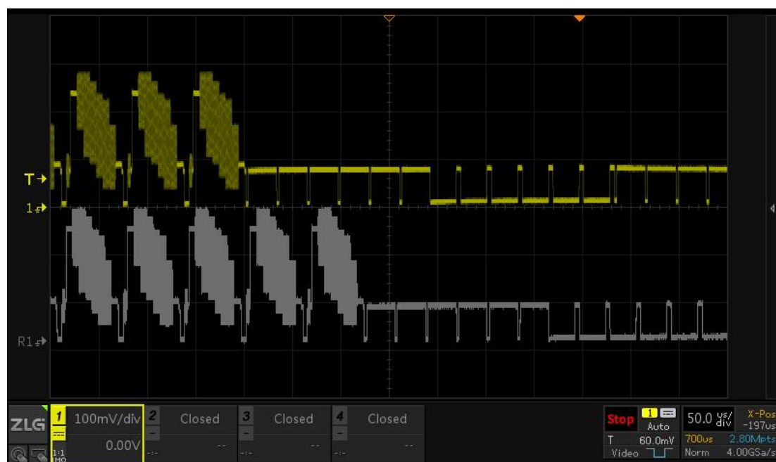
图 21.13 波形对比分析
