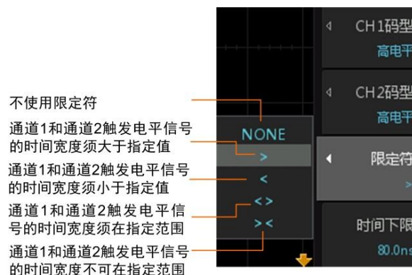
图 10.46 限定符设置说明
