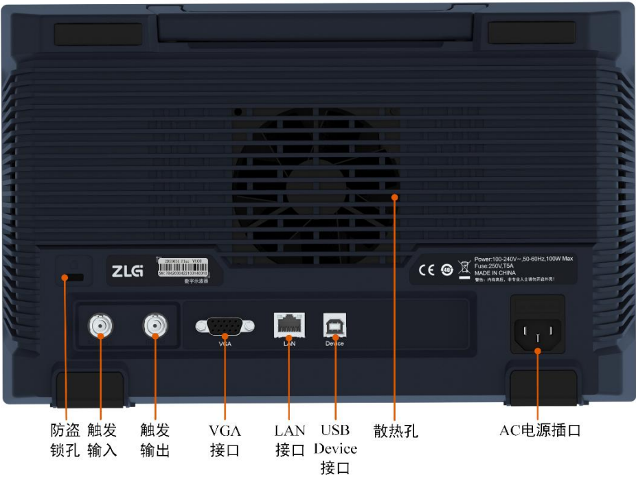
图 5.9 ZDS5054Pro 型示波器后面板
