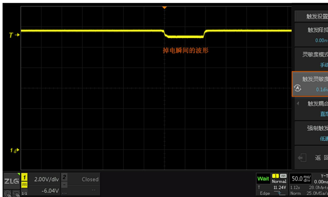
图 10.19 掉电波形稳定捕获
