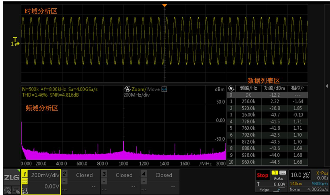
图 18.2 FFT 界面视图
