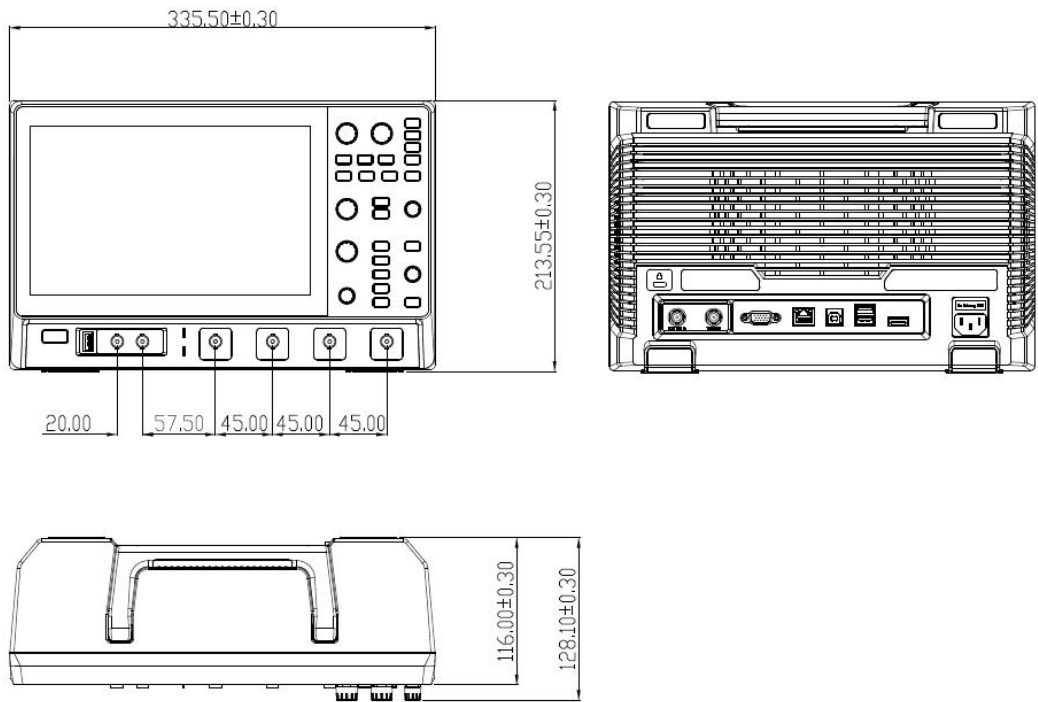
图 26.1 ZDS5000 示波器尺寸图
