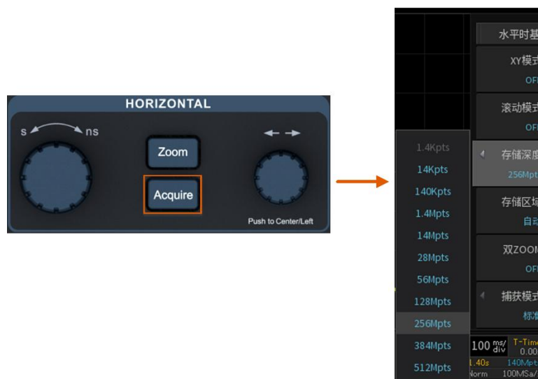
图 5.21 存储深度的调节
