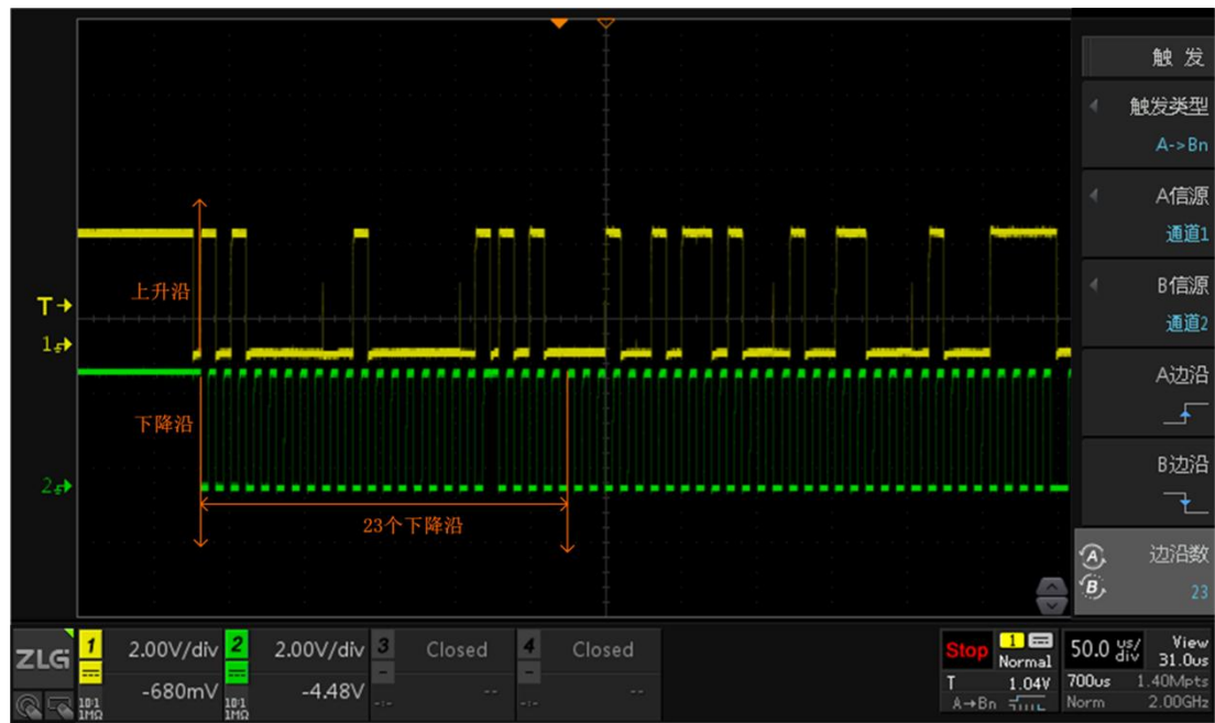
图 10.48 A->B 触发效果图
