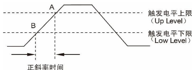
图 10.24 正斜率时间说明
