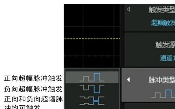
图 10.33 超幅触发的脉冲类型
