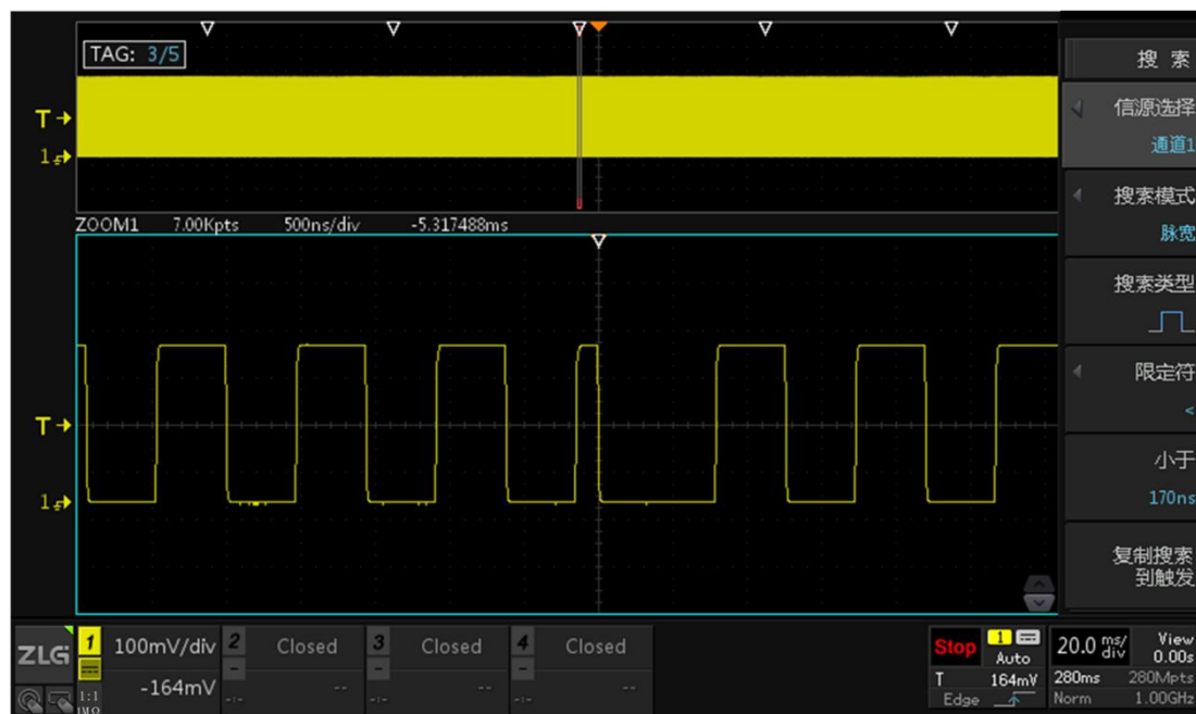
图 13.6 搜索结果放大
