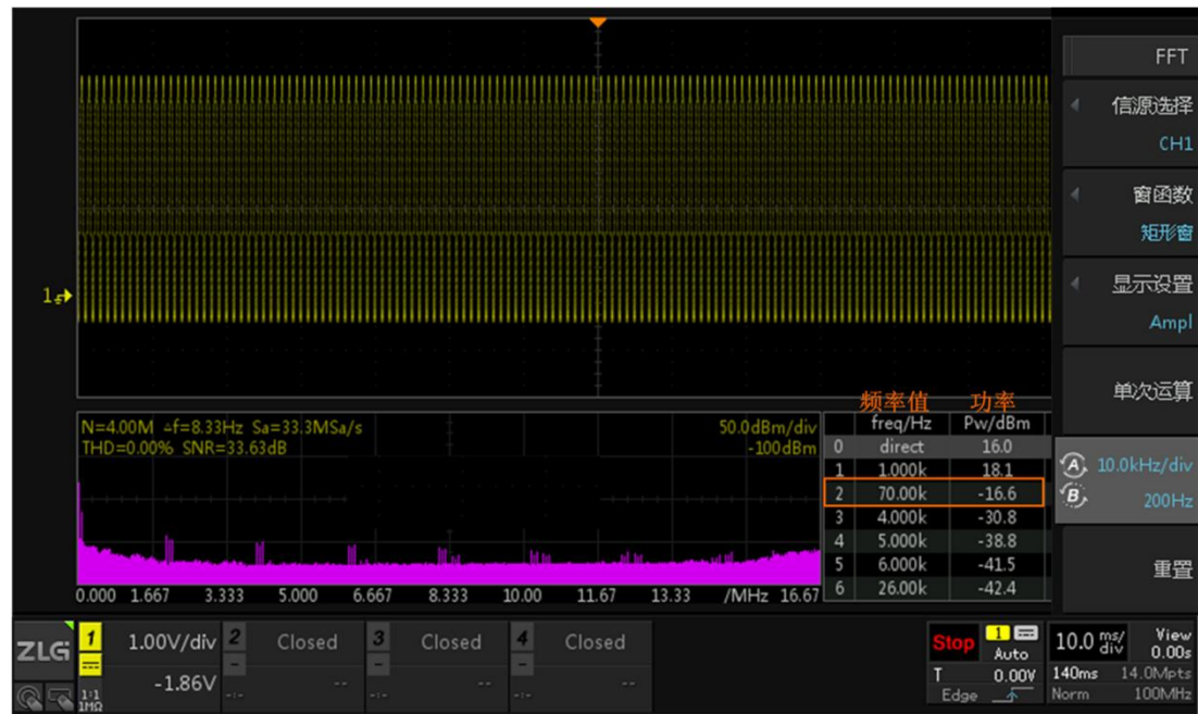
图 18.9 FFT 分析结果
