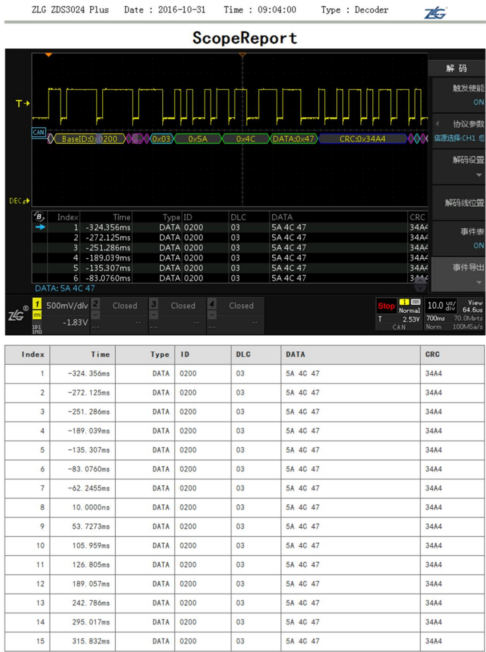
图 22.18 解码事件表报表实例
