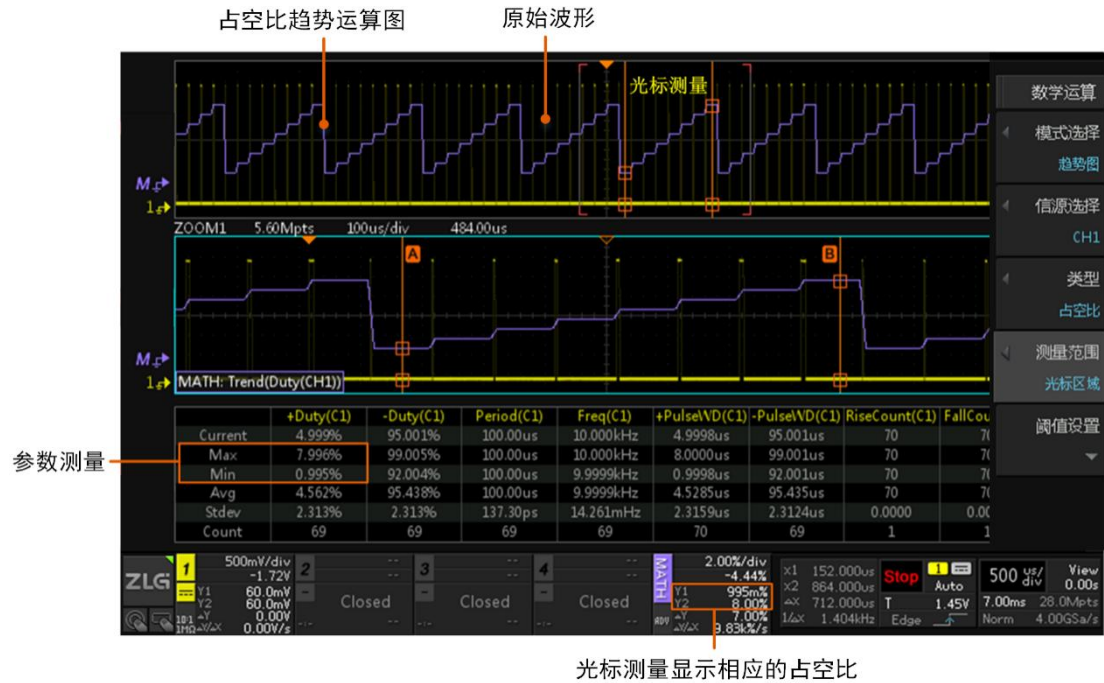
图 17.11 趋势运算界面
