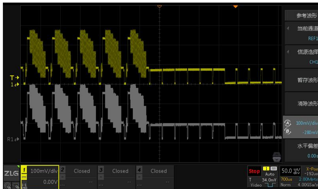
图 21.12 参考波形垂直方向调节
