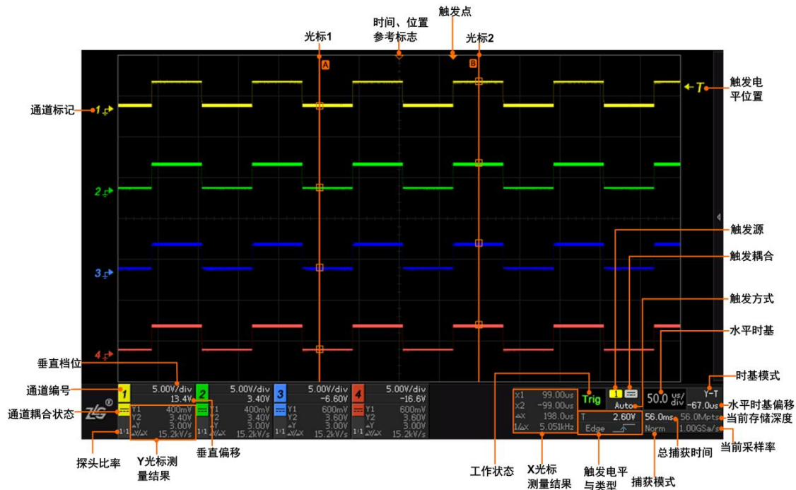
图 5.17 面板组件
