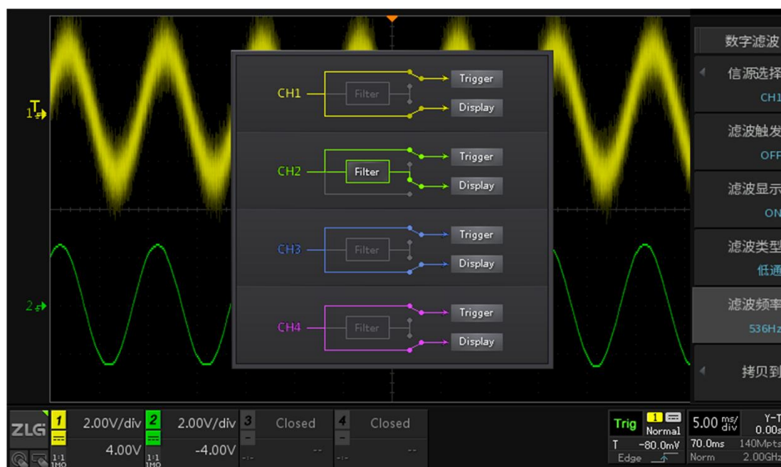
图 16.5 噪声滤波设置
