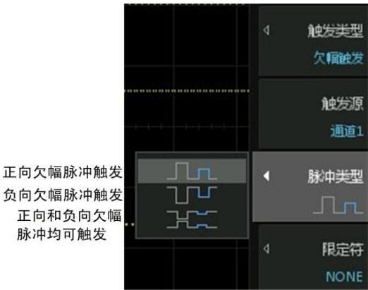
图 10.29 欠幅触发的脉冲类型
