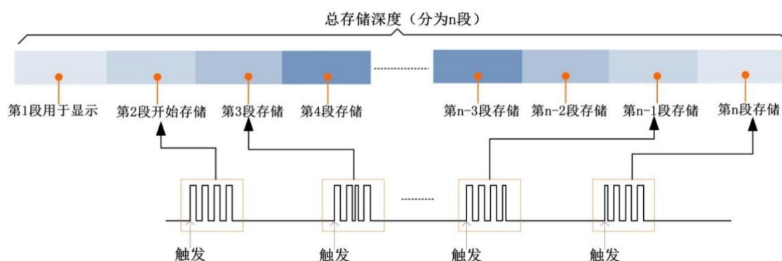
图 19.1 分段存储结构图
