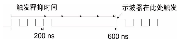
图 10.13 触发释抑时间设置
