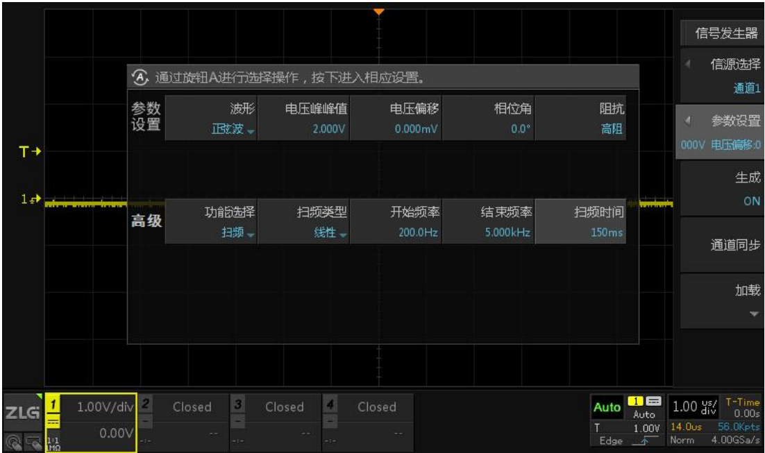
图 20.4 扫频参数设置
