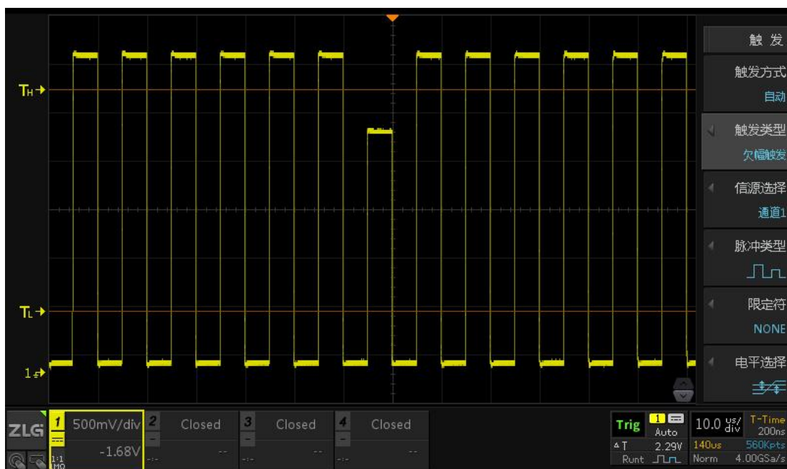
图 10.10 欠幅触发
