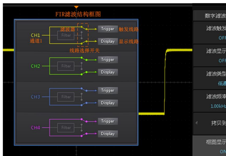
图 16.1 FIR 滤波界面
