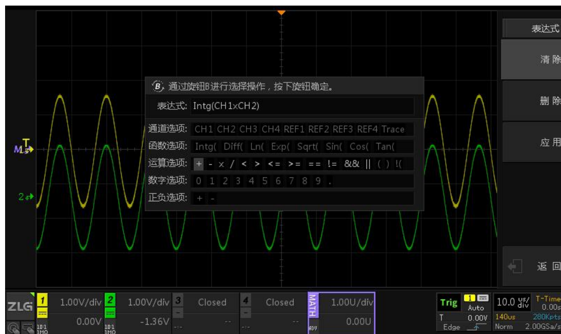
图 17.8 能量损耗表达式
