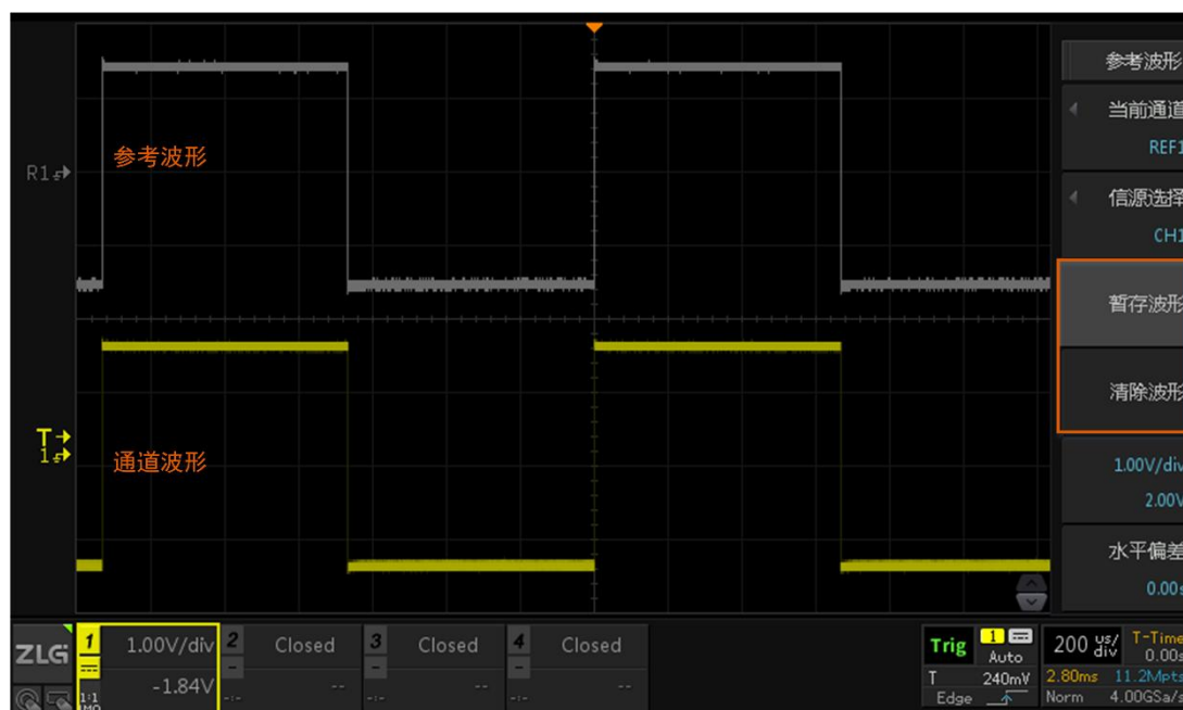
图 21.5 参考波形显示与对比
