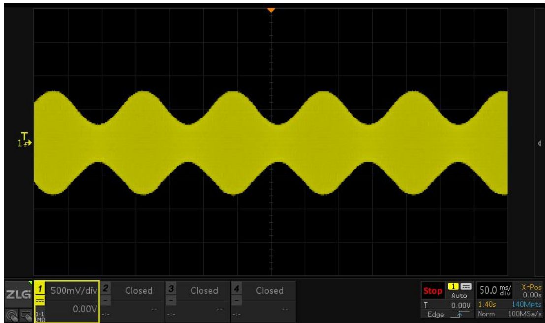
图 20.7 调制效果图
