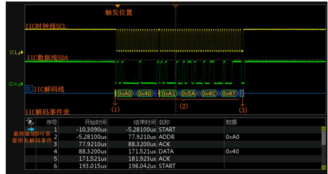
图 15.1 解码功能示意（ZDS5054Pro 型）
