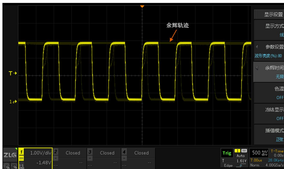
图 8.2 无限余辉显示效果
