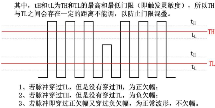
图 10.32 欠幅原理解析
