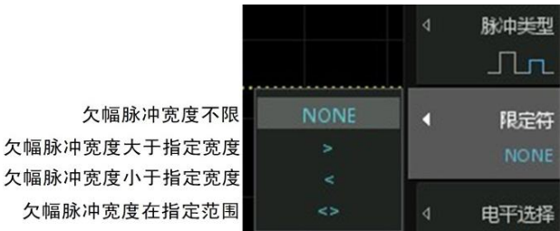
图 10.30 欠幅脉冲宽度限定
