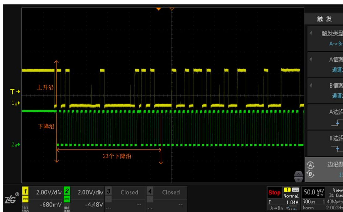
图 10.53 A->B 触发效果图
