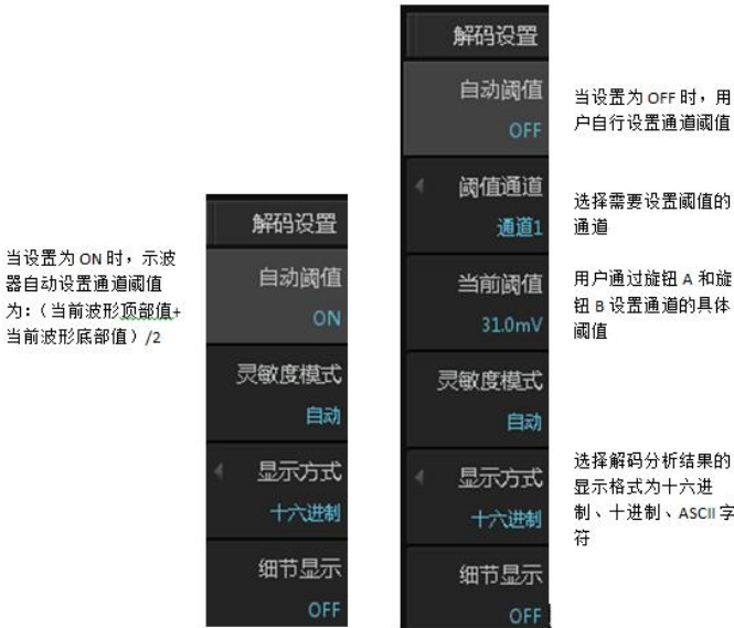
图 15.14 解码设置说明
