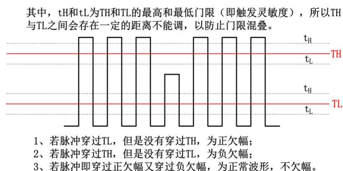
图 10.34 欠幅原理解析
