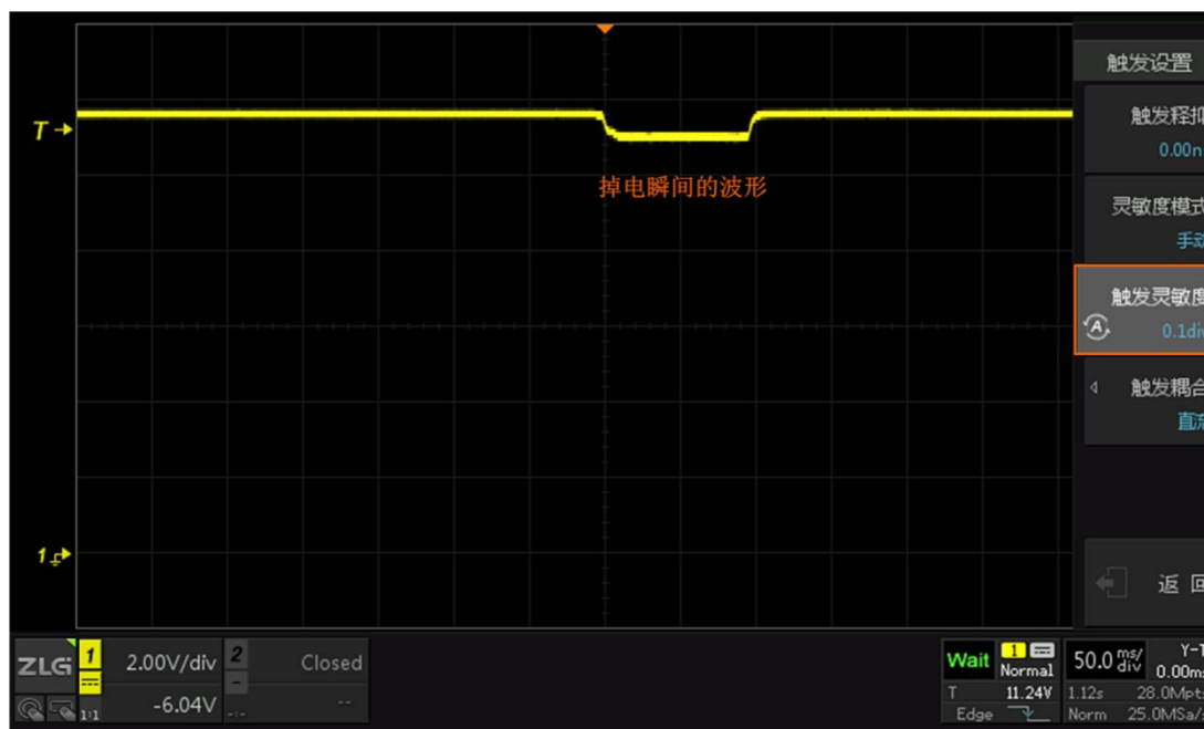
图 10.21 掉电波形稳定捕获
