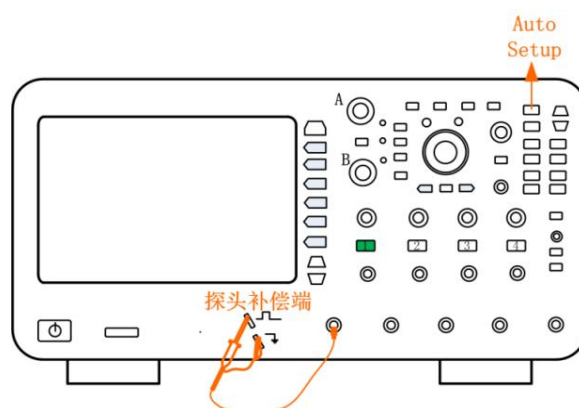
图 5.21 探头接线图
