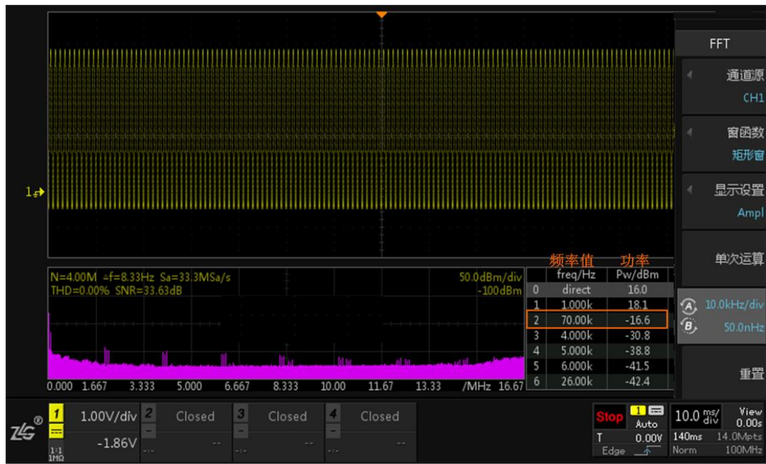
图 19.9 FFT 分析结果
