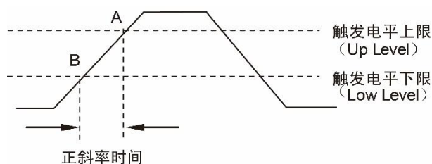
图 10.26 正斜率时间说明
