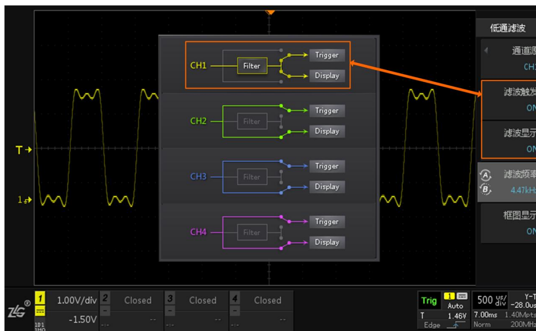
图 17.3 滤波触发和显示
