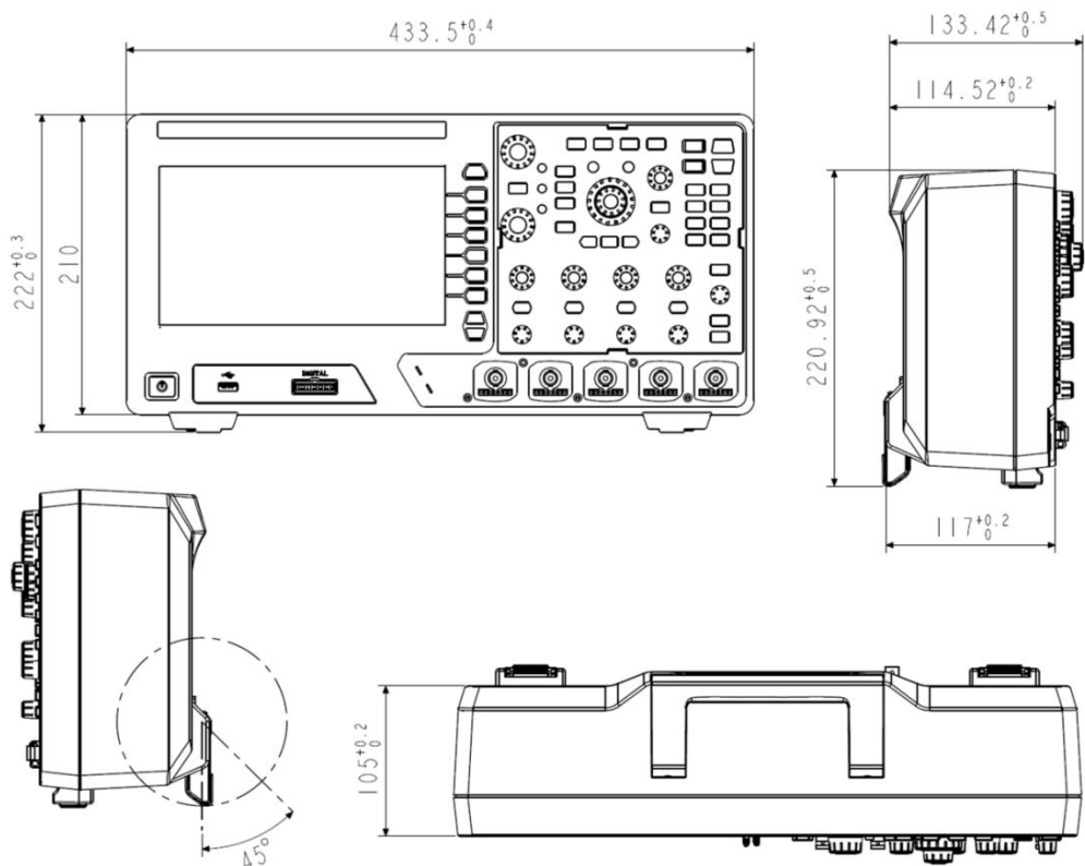
图 26.1 ZDS3000/4000 示波器尺寸图
