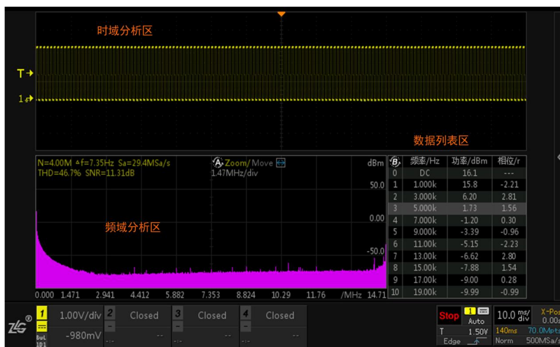
图 19.2 FFT 界面视图
