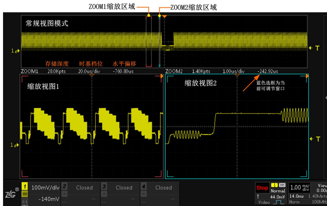
图 6.6 双 ZOOM 显示模式
