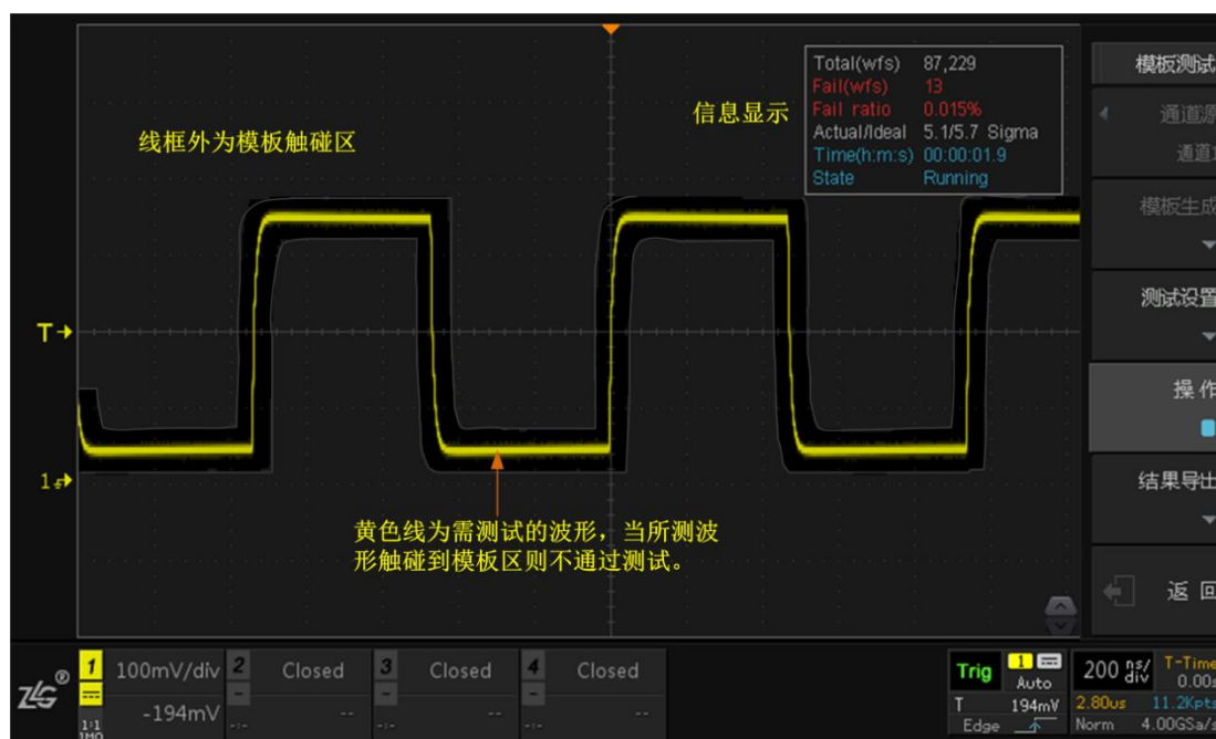
图 24.2 模板测试界面
