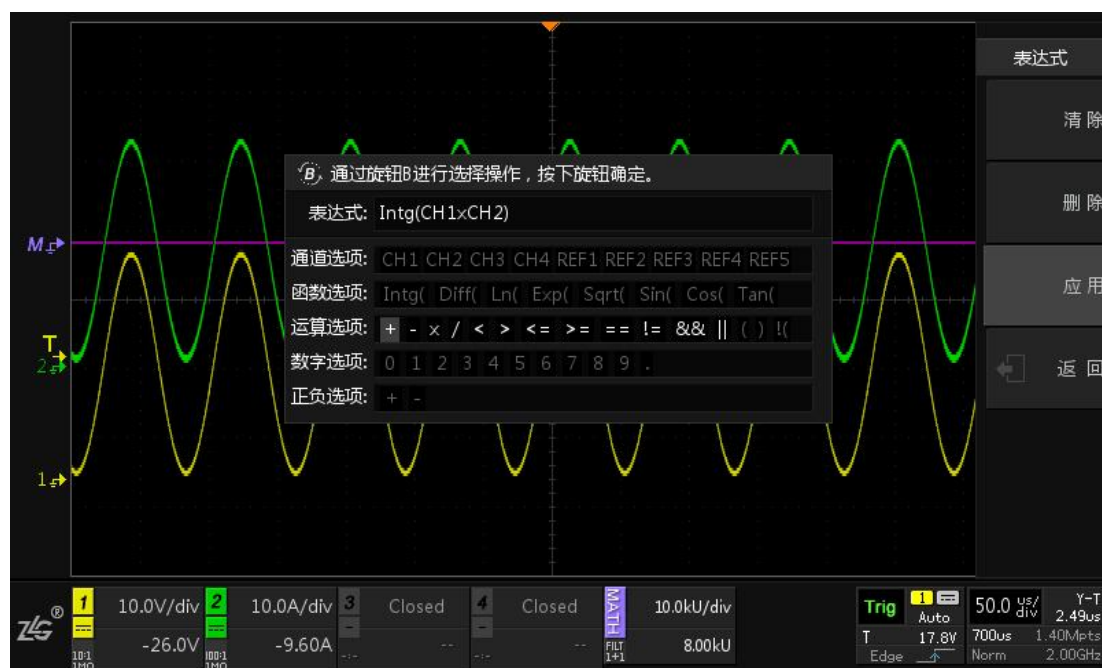
图 18.8 能量损耗表达式
