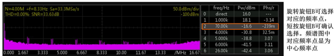
图 19.10 FFT 频谱表操作
