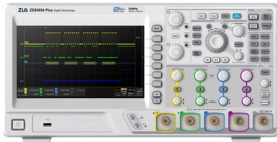
图 3.1 ZDS4054 Plus 示波器面板
