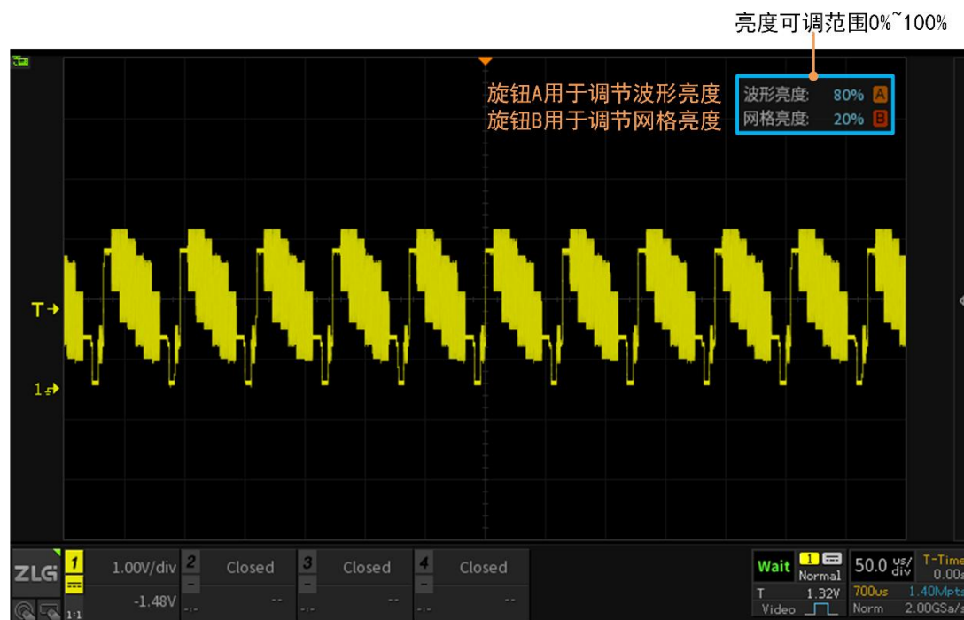
图 7.2 波形亮度调节界面
