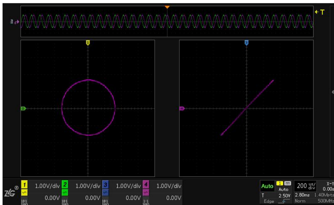
图 9.9 4 通道示波器 X-Y 模式
