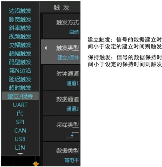
图 10.43 触发类型
