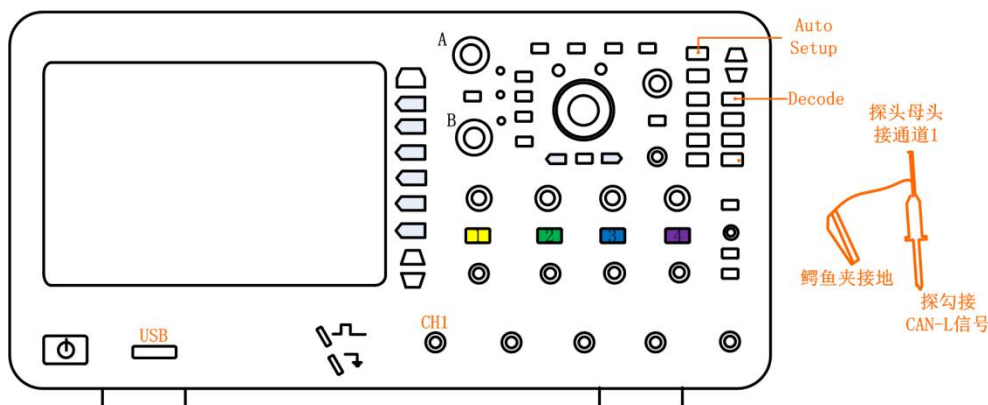
图 15.4 接入 CAN-L 信号
