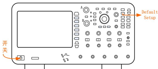
图 5.2 默认设置
