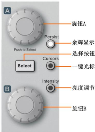
图 5.11 多功能旋钮区面板
