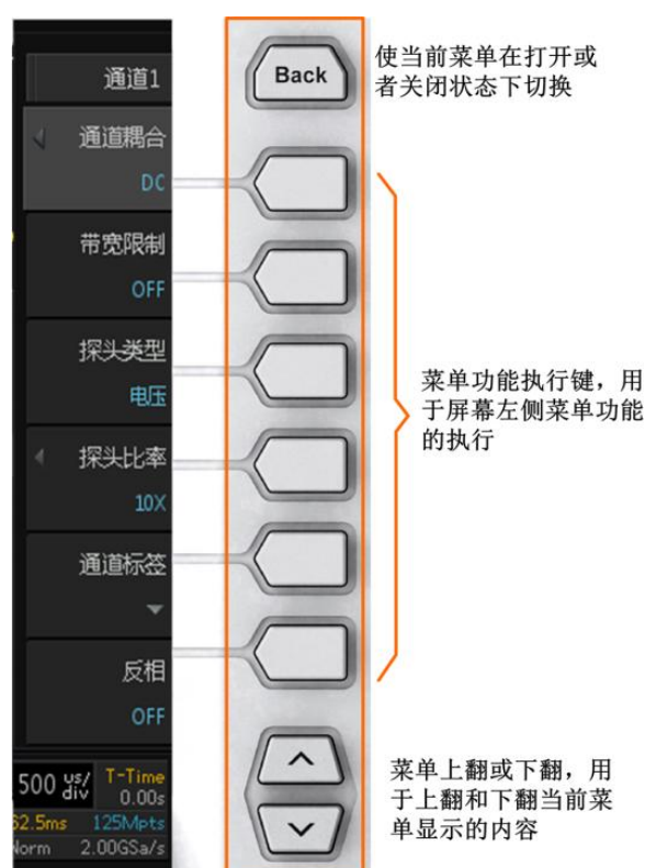
图 5.10 软键区
