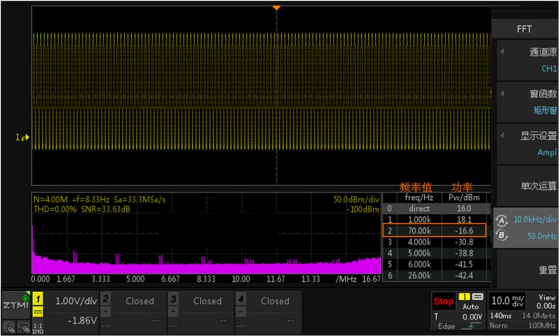
图 18.10 FFT 分析结果
