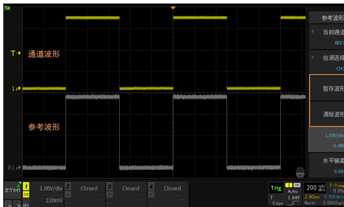
图 20.5 参考波形显示与对比
