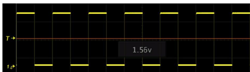
图 10.2 触发电平线
