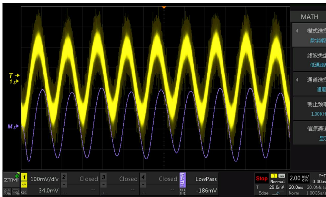
图 17.15 滤波后的波形
