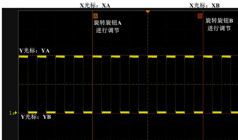
图 11.1 X 型光标和 Y 型光标
