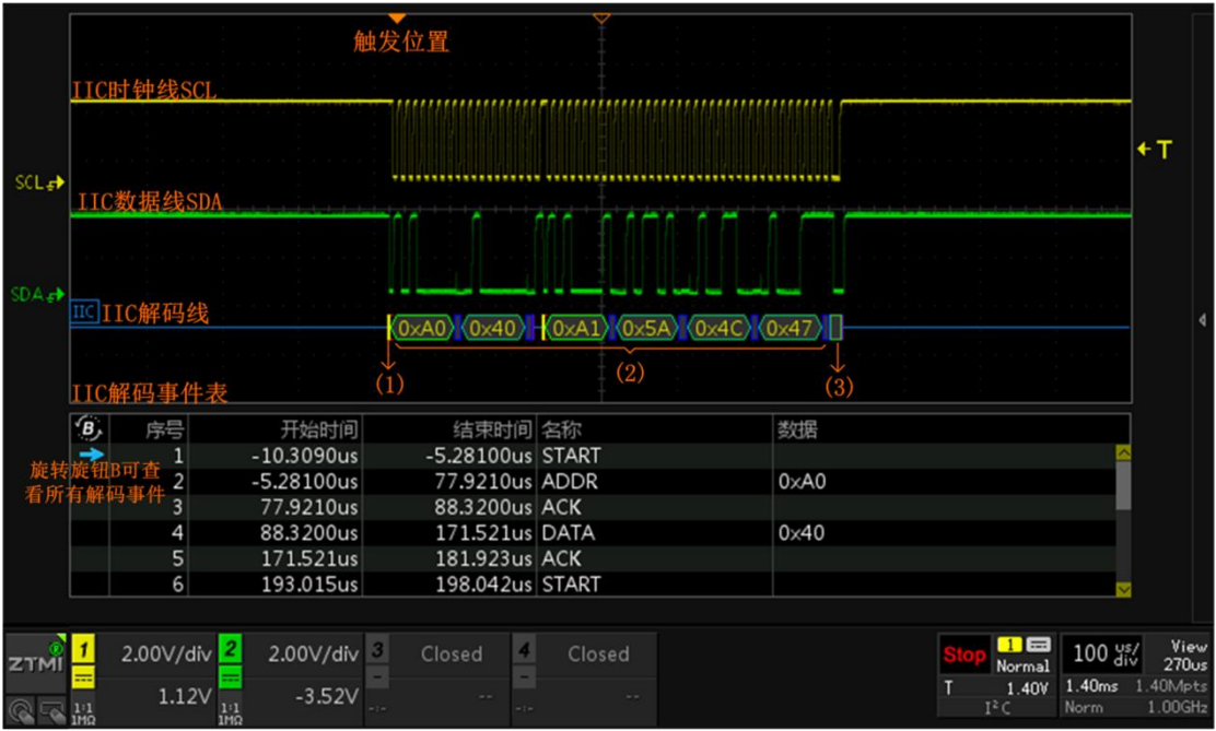
图 15.1 解码功能示意（ZDS3024D 型）
