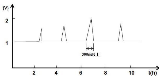
图 19.9 测试波形
