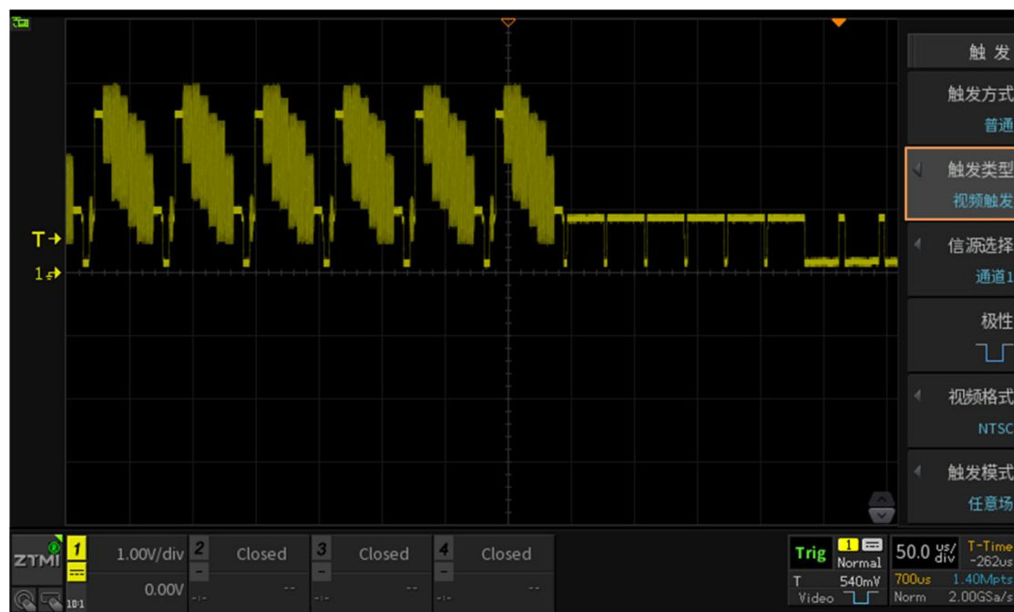
图 20.10 视频触发
