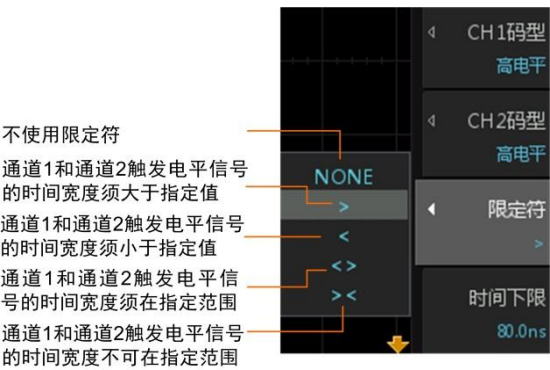
图 10.49 限定符设置说明
