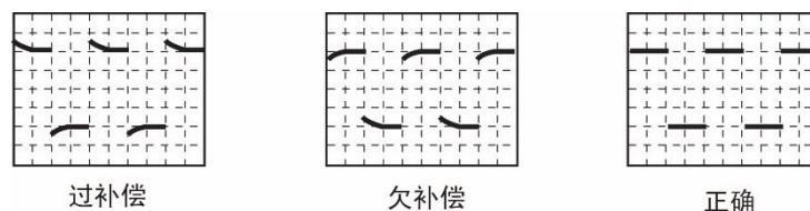
图 5.4 探头补偿信号
