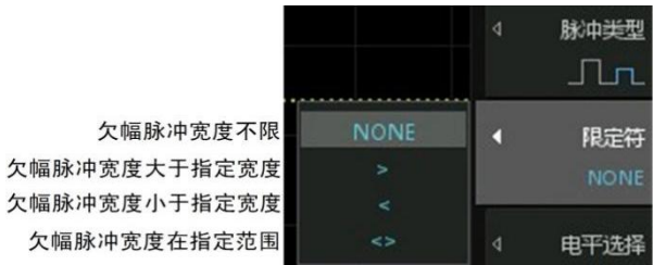
图 10.32 欠幅脉冲宽度限定
