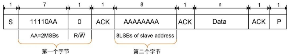
图 15.23 10 位寻址
