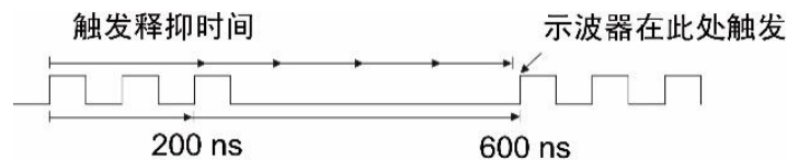
图 10.15 触发释抑时间设置
