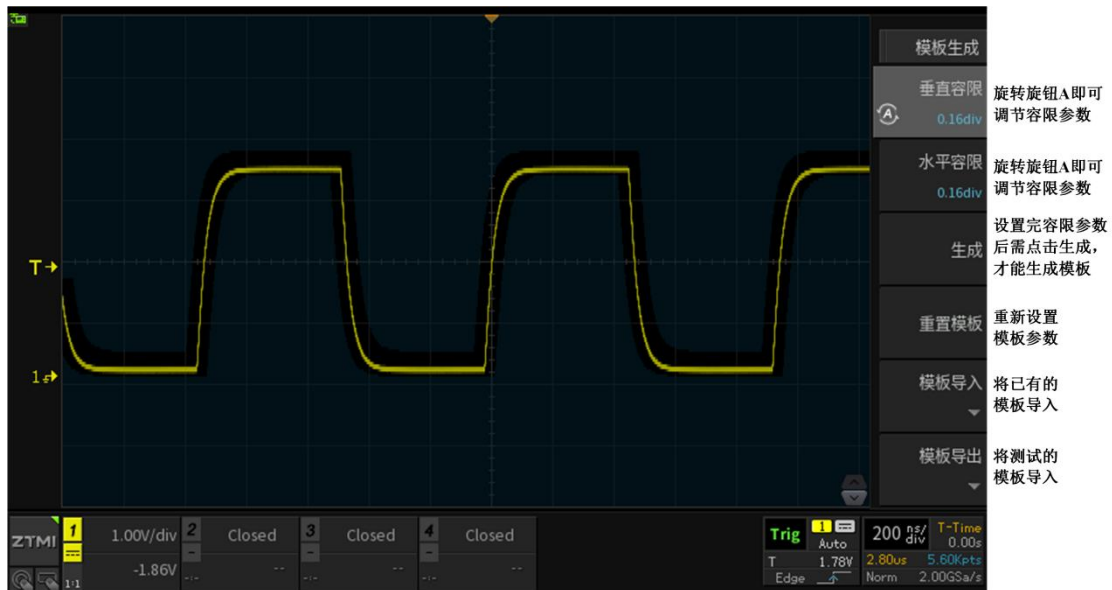
图 23.4 模板生成界面
