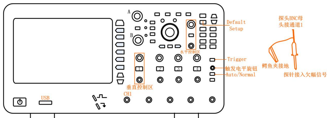
图 10.9 欠幅信号的输入
