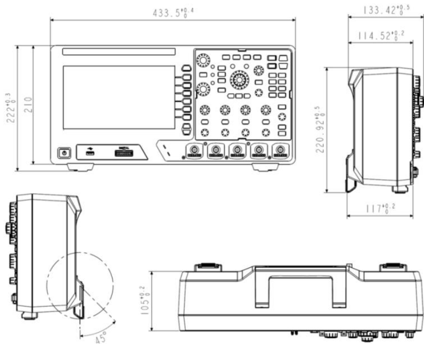
图 25.1 ZDS3000C/ZDS3000D/ZDS3000E 系列示波器尺寸图
