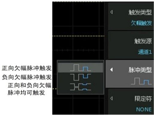
图 10.31 欠幅触发的脉冲类型
