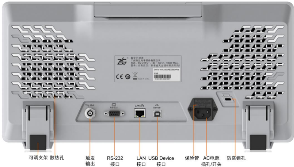
图 5.9 ZDS3024D 型示波器后面板
