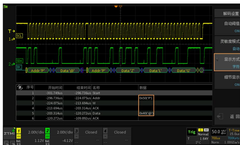
图 15.29 字符显示
