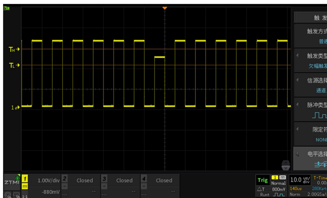
图 10.10 欠幅触发
