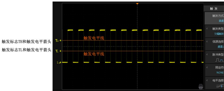
图 10.3 TH 和 TL 触发标志
