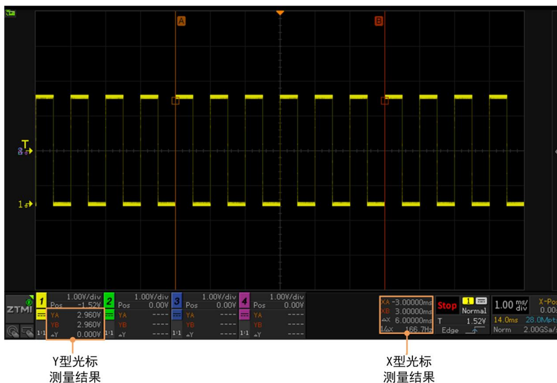
图 11.3 光标测量结果
