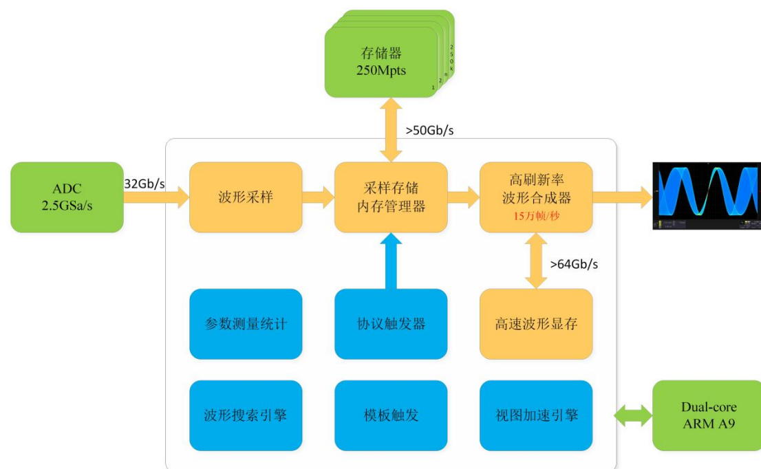
图 3.2 ZDS3000D 系列示波器系统框图
