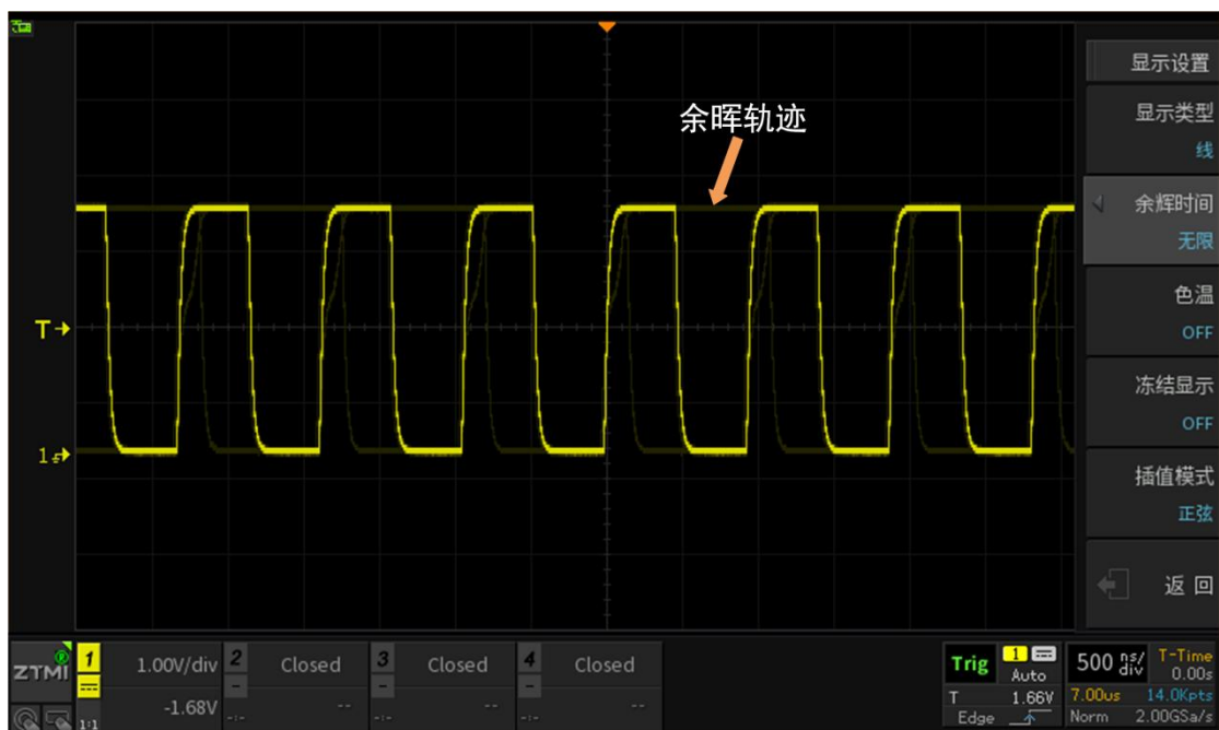
图 8.3 无限余辉显示效果
