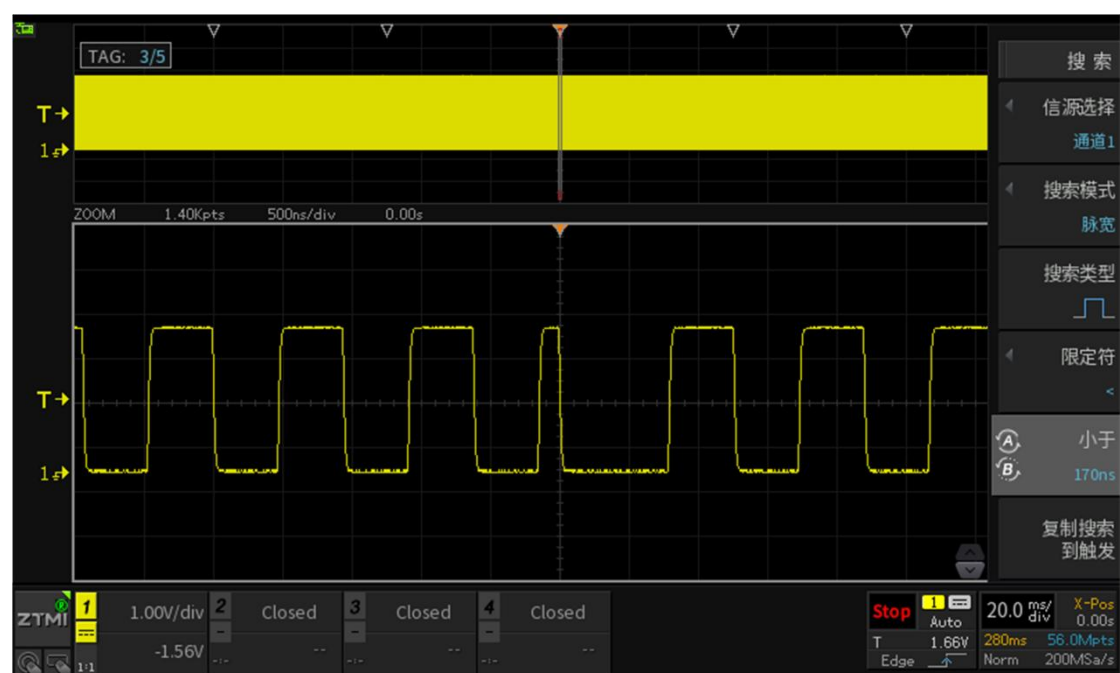
图 13.8 搜索结果放大
