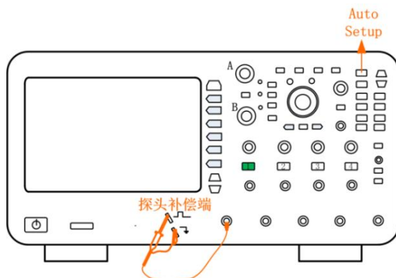
图 5.3 探头连接
