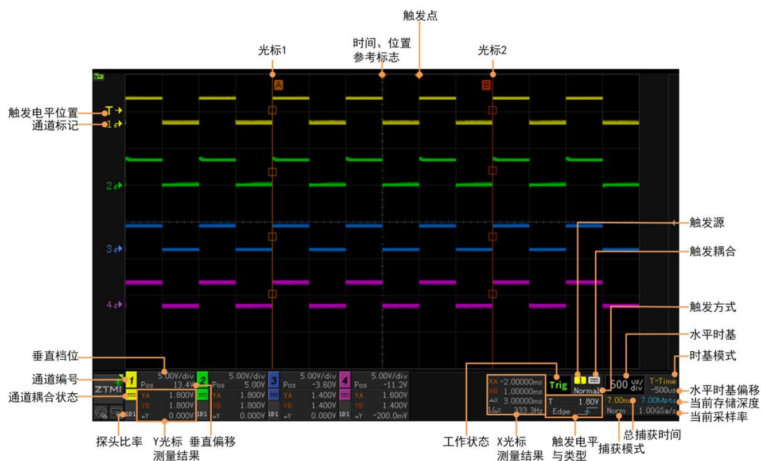
图 5.19 面板组件
