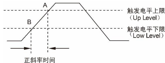
图 10.26 正斜率时间说明
