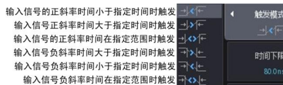
图 10.25 触发模式设置
