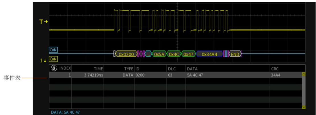
图 15.17 事件表
