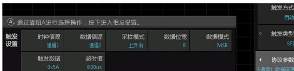
图 10.54 SPI 触发协议参数
