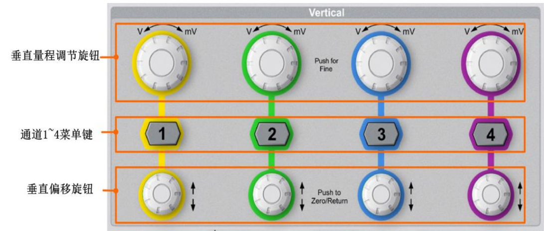
图 5.17 垂直控制区
