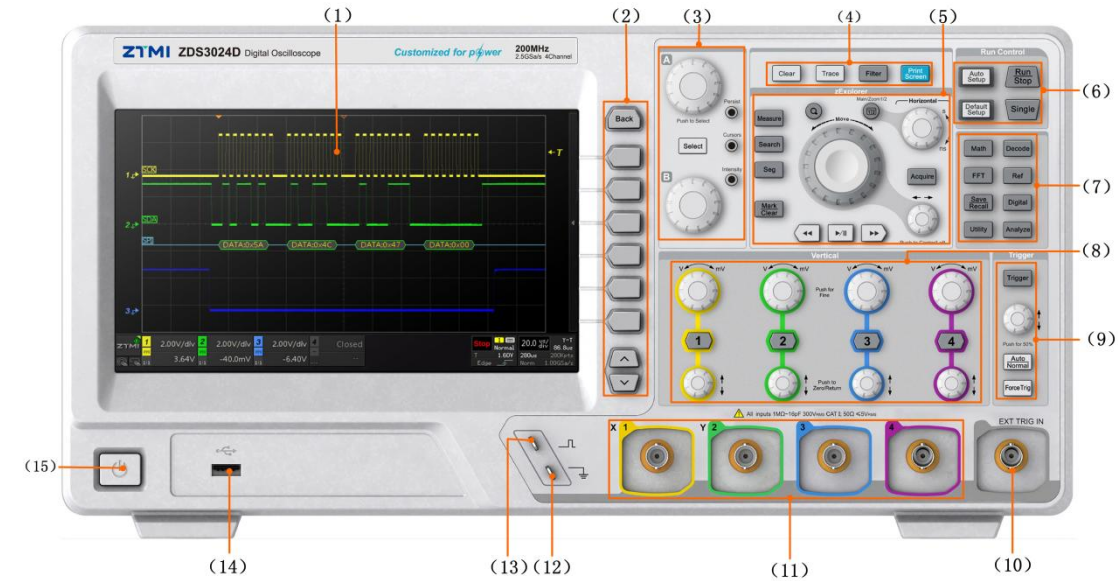
图 5.8 ZDS3024D 型台式示波器前面板
