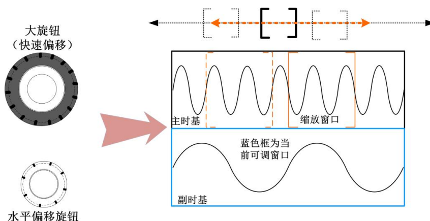
图 6.6 波形/缩放窗口偏移
