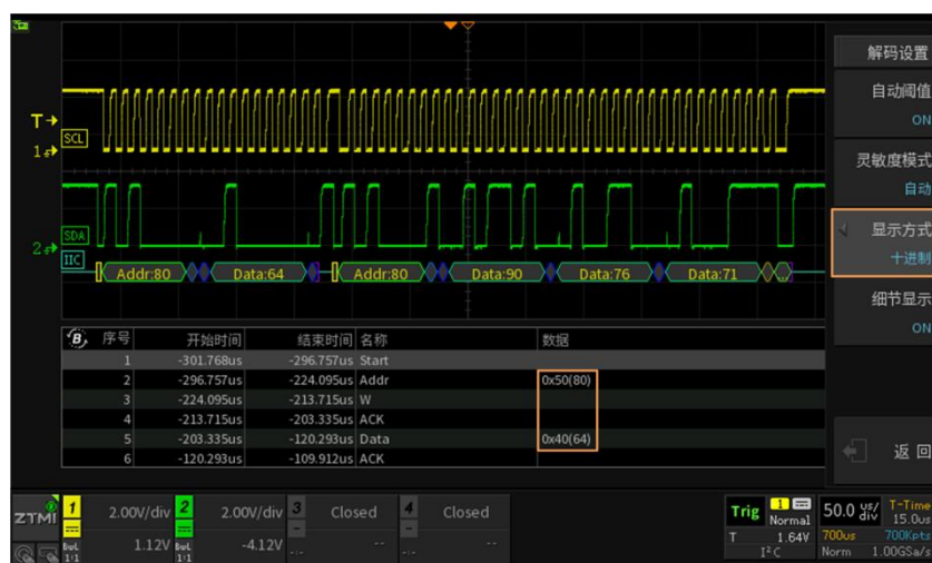
图 15.28 十进制显示
