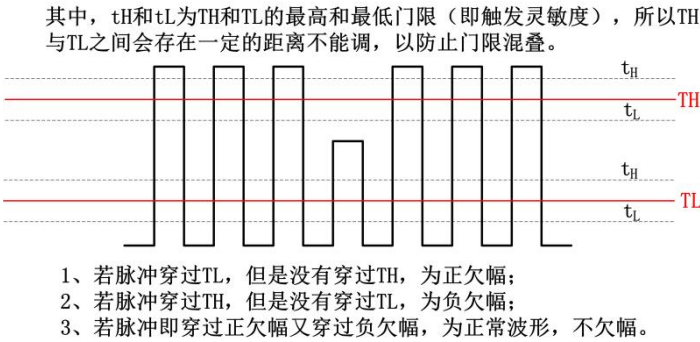
图 10.34 欠幅原理解析
