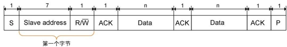
图 15.22 7 位寻址
