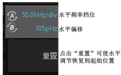
图 18.6 水平调节
