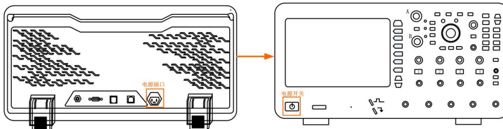
图 5.1 上电操作
