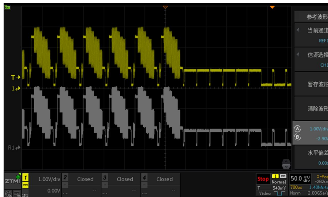
图 20.12 参考波形垂直方向调节
