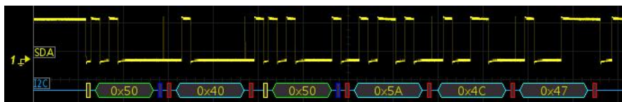
图 15.30 细节显示
