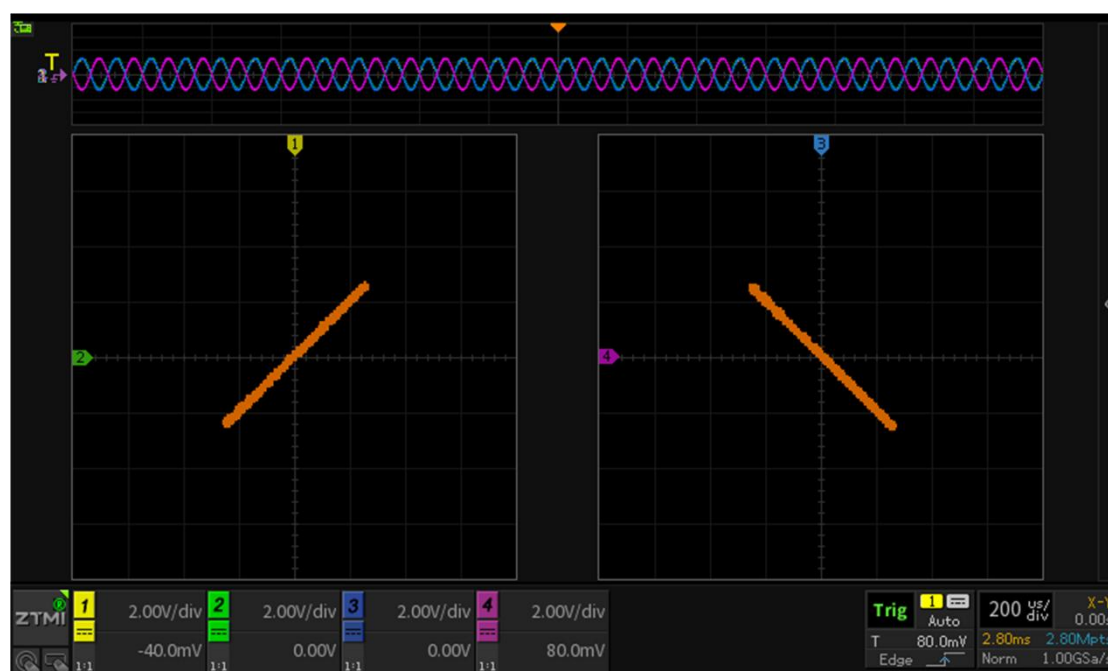
图 9.10 45°斜线
