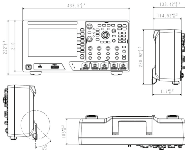
图 4.1 ZDS3000C/ZDS3000D/ZDS3000E 系列示波器尺寸图
