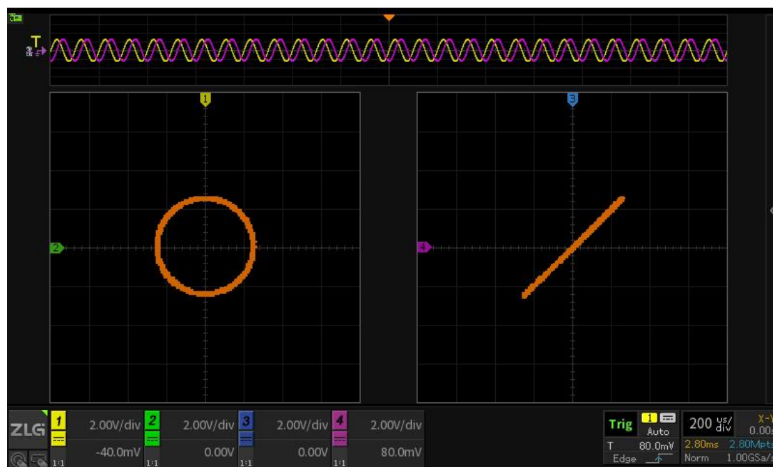
图 9-9 4 通道示波器 X-Y 模式
