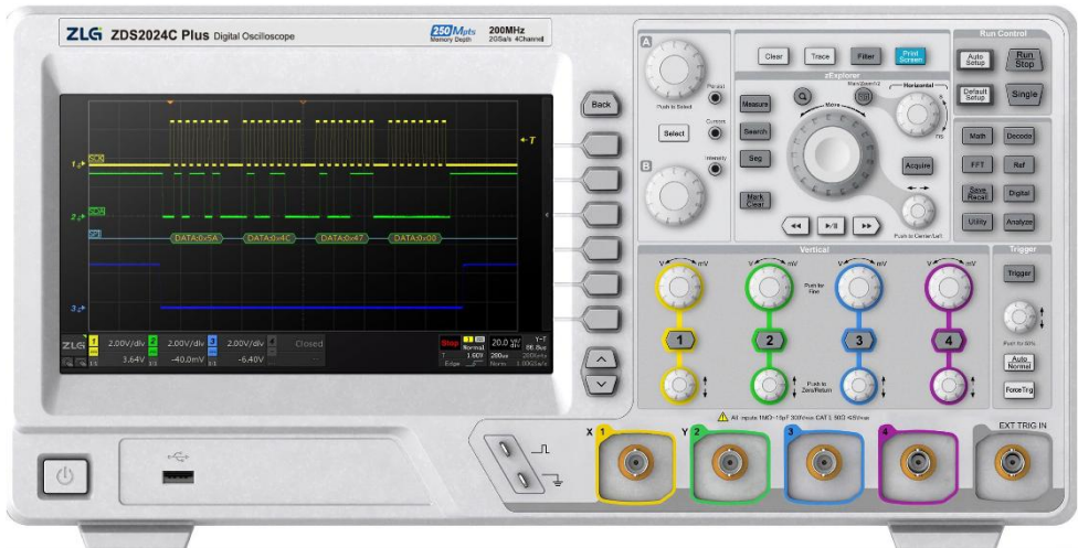
图 3-1 ZDS2024C Plus 示波器面板
