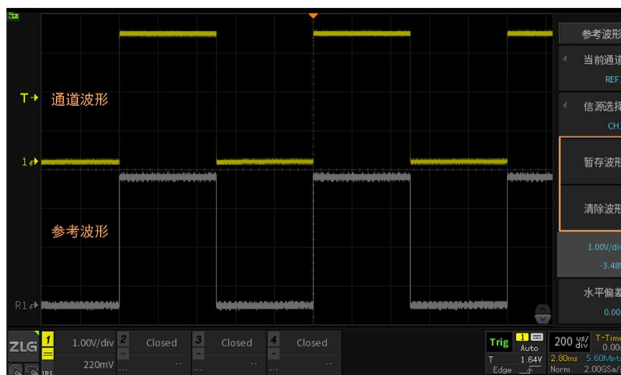
图 20-5 参考波形显示与对比
