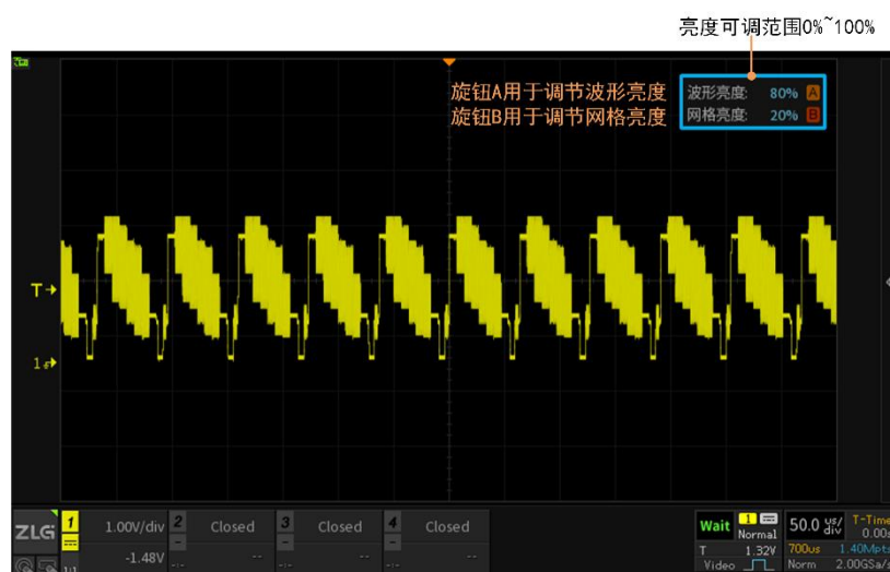
图 7-2 波形亮度调节界面
