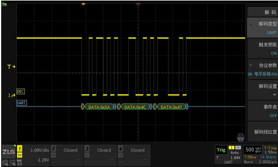
图 15-36 ZDS2000C 系列示波器的 UART 信号
