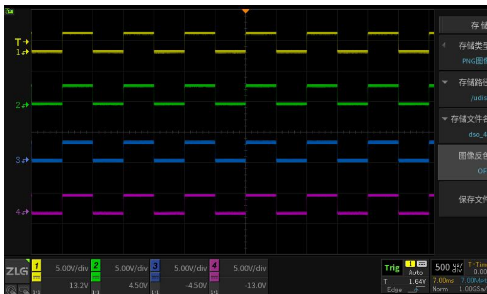
图 21-13 图像反相为“OFF”
