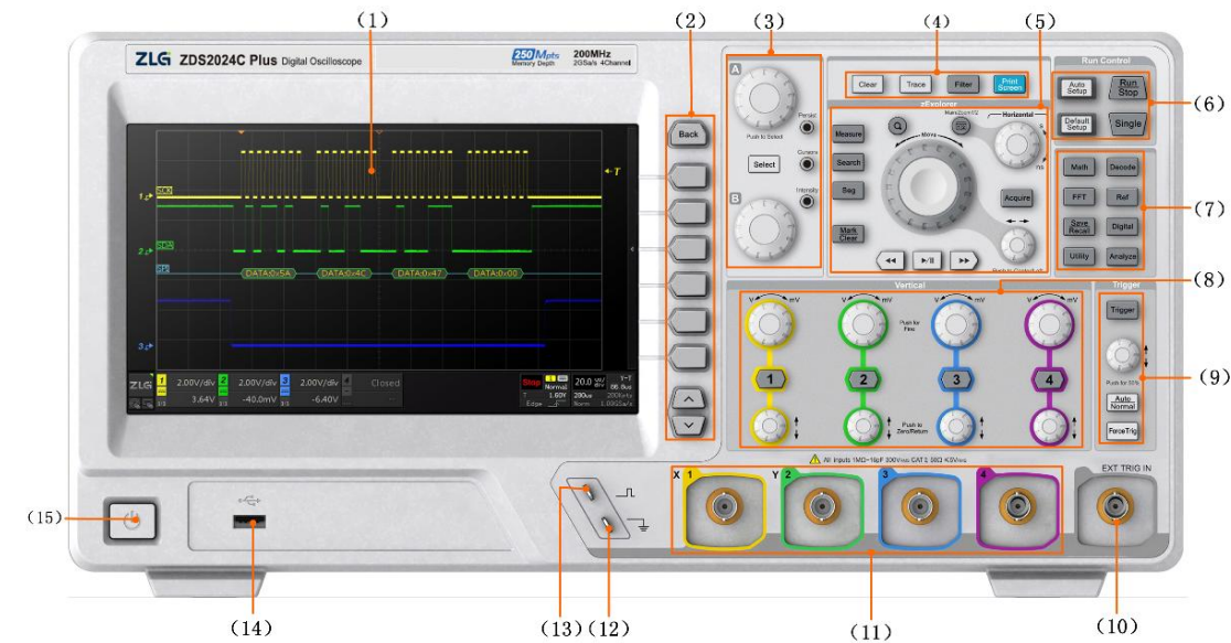
图 5-8 ZDS2024C Plus 型台式示波器前面板
