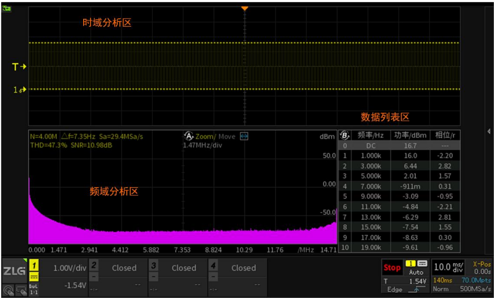
图 18-2 FFT 界面视图
