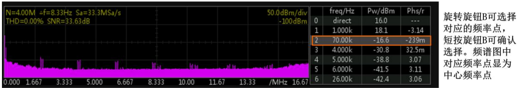
图 18-11 FFT 频谱表操作
