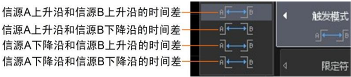
图 10-39 设置触发模式
