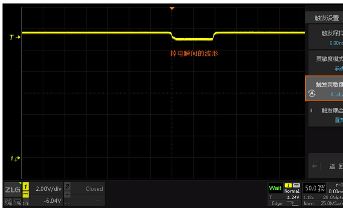
图 10-21 掉电波形稳定捕获
