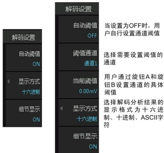
图 15-14 解码设置说明
