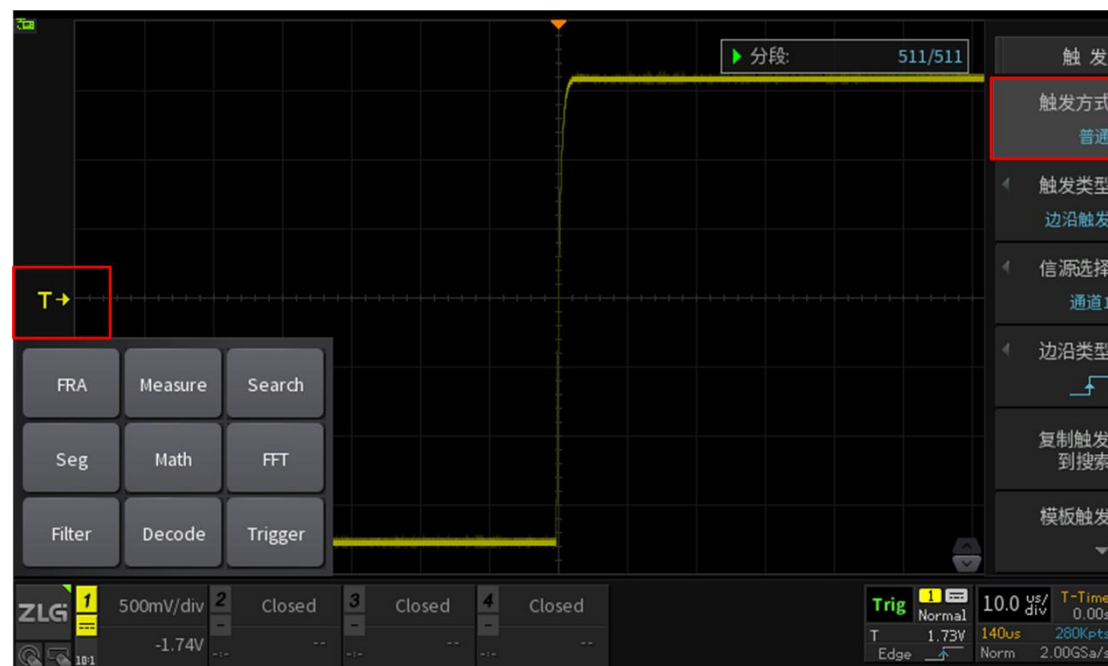
图 19-3 触发方式设置
