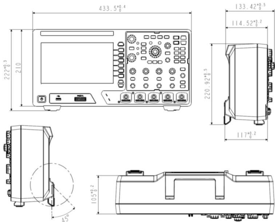
图 24-1 ZDS2000C 示波器尺寸图
