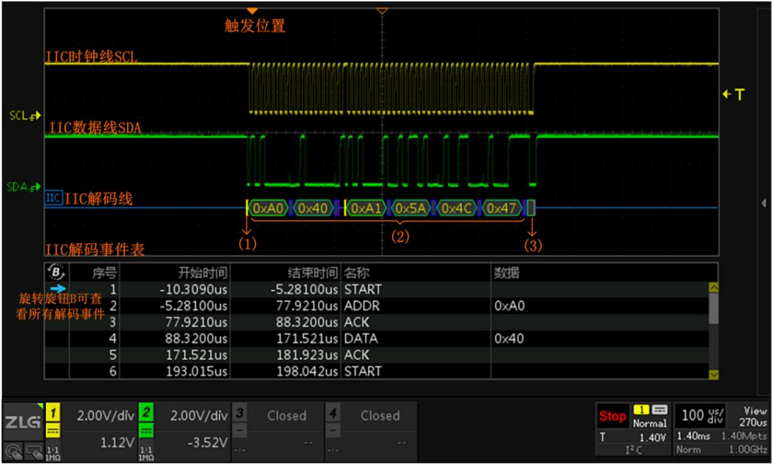
图 15-1 解码功能示意（ZDS2024C Plus 型）
