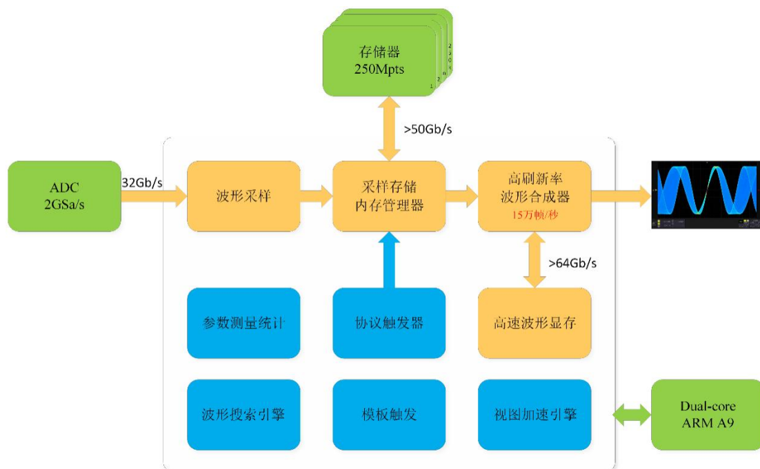
图 3-2 ZDS2000C 系列示波器系统框图
