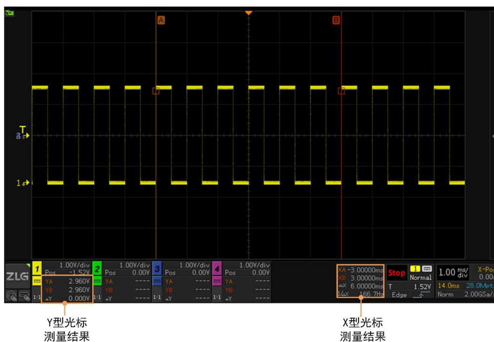
图 11-3 光标测量结果
