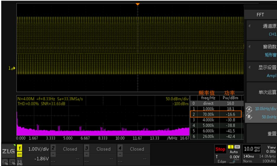
图 18-10 FFT 分析结果
