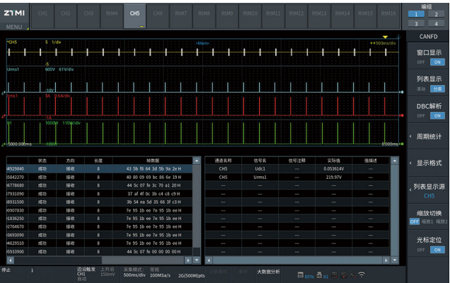
电压、电流、CAN信号同步分析
