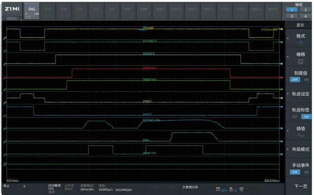
充电桩时序分析测试图
