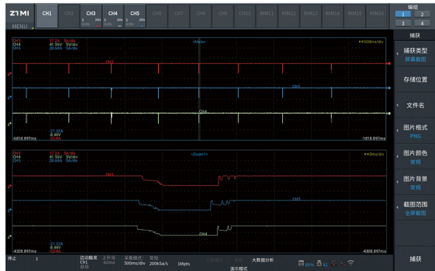
时序分析-吸合时间、释放时间分析
