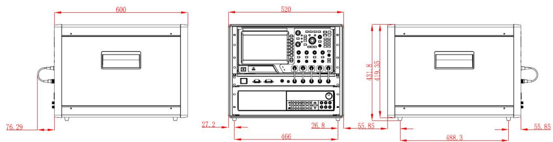
图 6.1 CANDT 尺寸图
