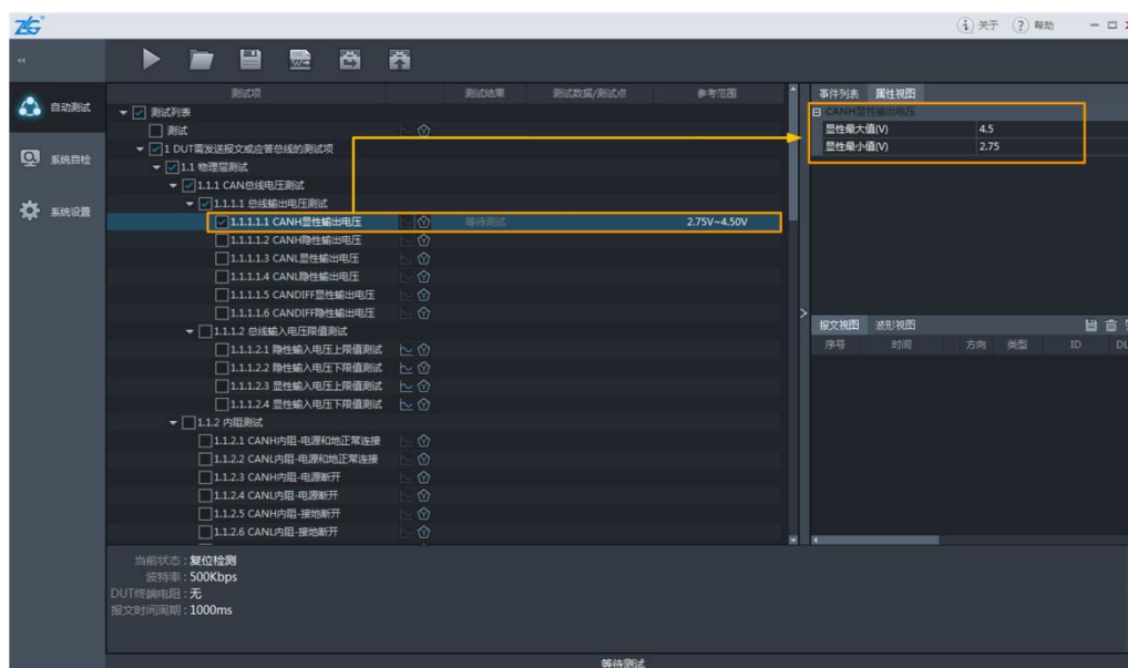
图 4.9 测试项参考范围设置
